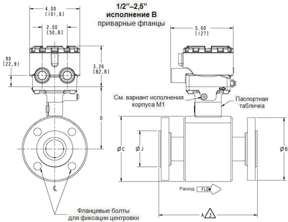
Рисунок 9. Фланцевый датчик расхода 8705-M, типоразмер от 0,5 дюйма до 2,5 дюйма (DN 15–65 мм), приварной фланец, для работы под низким давлением (P < класс 300)
