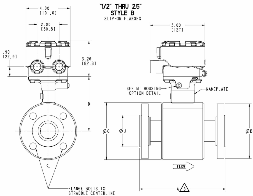
Рисунок 14. Фланцевый датчик 8705-М, типоразмер от 1/2 дюйма до 24 дюймов (DN 15–600 мм), приварной фланец, для работы под высоким давлением (P ≤ класс 900)
