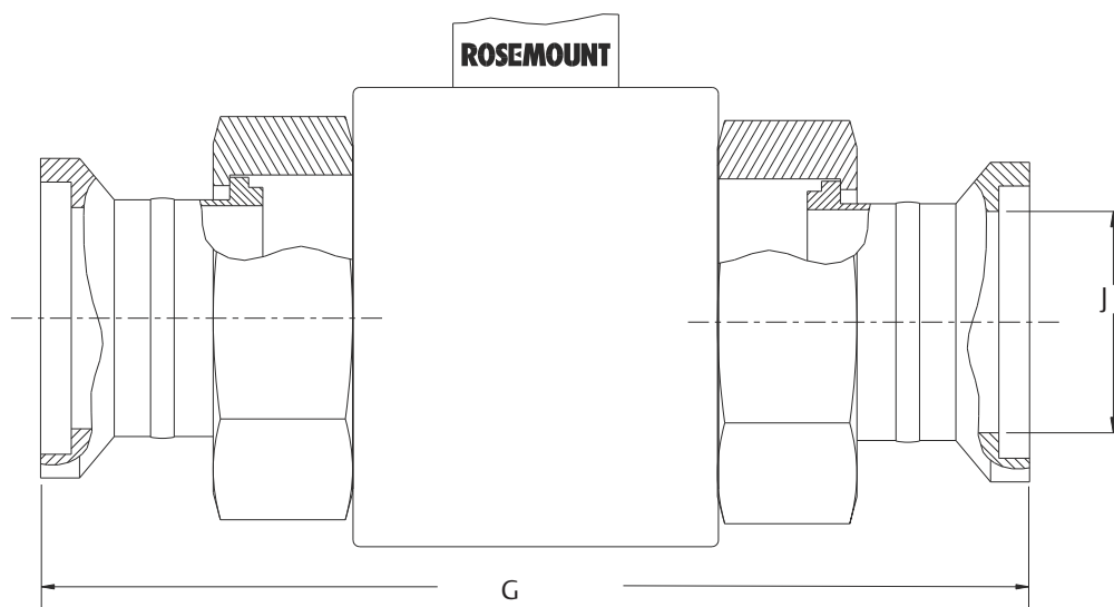
Рисунок 27. Датчик гигиенического (санитарного) исполнения 8721, фитинг Cherry Burrell I-Line
