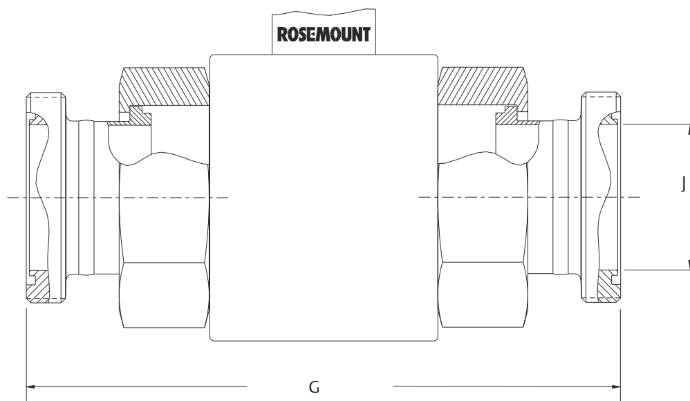
Рисунок 26. Датчик гигиенического (санитарного) исполнения 8721, SMS1145
