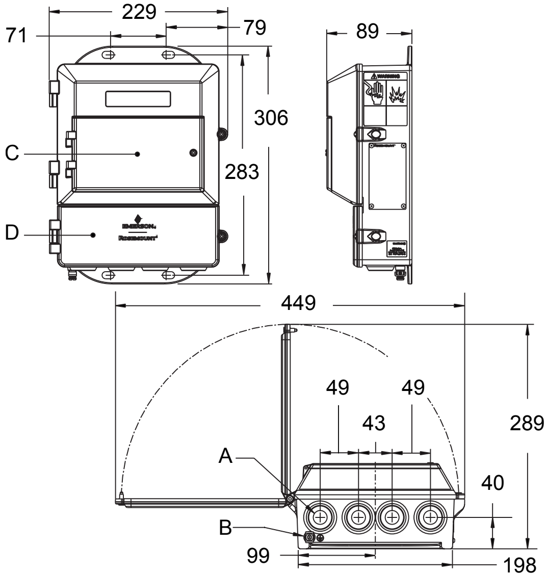
Рисунок 7. Размеры преобразователя 8712 для настенного монтажа
