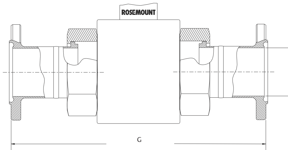
Рисунок 26. Датчик гигиенического (санитарного) исполнения 8721, SMS1145
