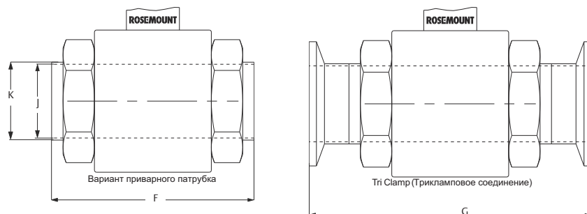
Рисунок 21. Приварной патрубок и триклампное соединение сенсора 8721 гигиенического (санитарного) исполнения
