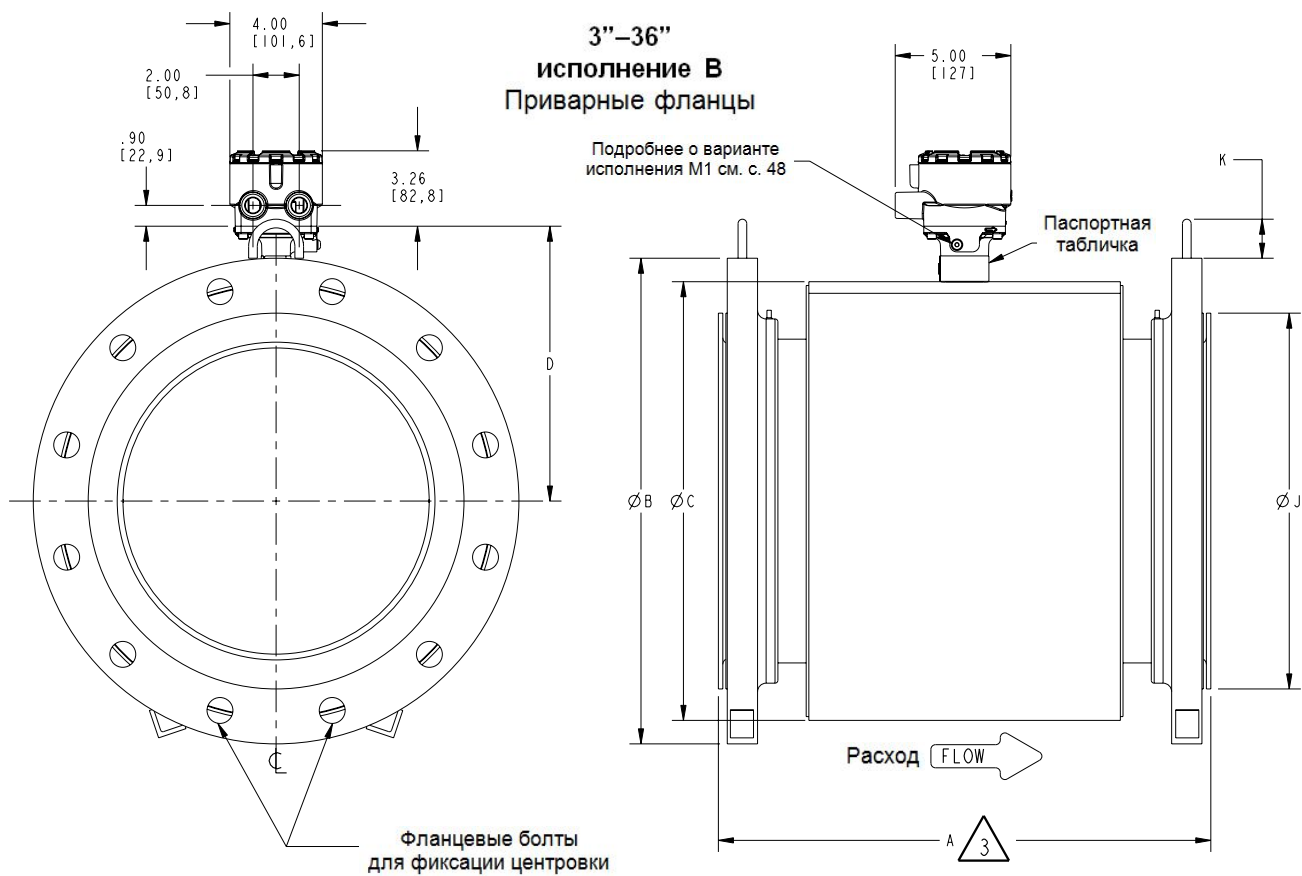
Рисунок 10. Фланцевый датчик 8705-М, типоразмер от 3 дюймов до 36 дюймов (DN 80–900 мм), приварной фланец, для работы под низким давлением ( P \leq класс 300)
