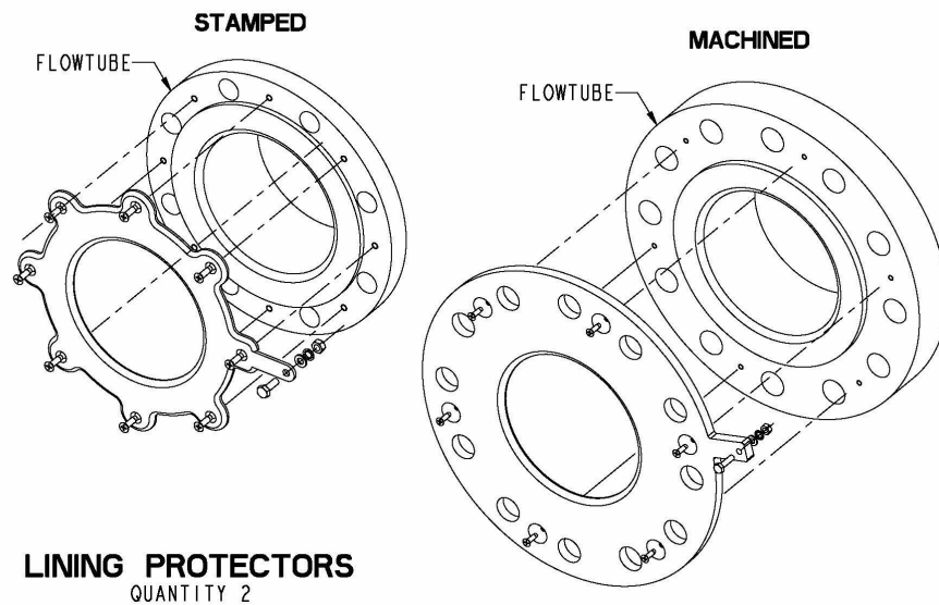
Рисунок 17. Фланцевый датчик 8705-М, типоразмер от 1/2 дюйма до 36 дюймов (DN 15–900 мм), протекторы футеровки (P ≤ класс 900)
