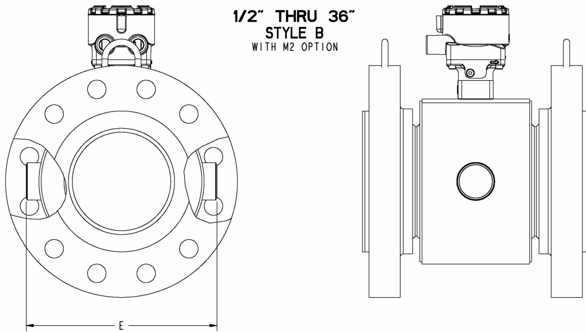
Рисунок 16. Фланцевый датчик 8705-М, типоразмер от 1/2 дюйма до 36 дюймов (DN 15–900 мм), корпус катушки M2/M4, (P ≤ класс 2500)
