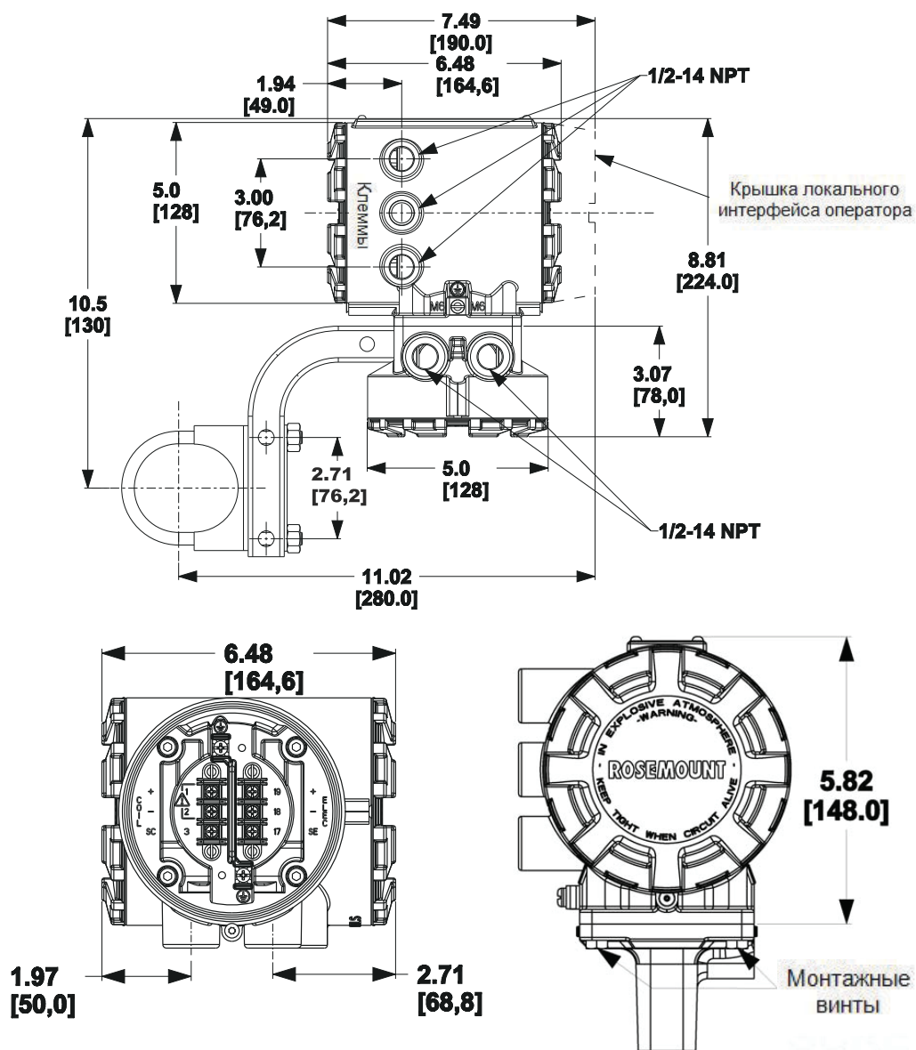
Рисунок 8. Размеры преобразователя 8732 для полевого монтажа
