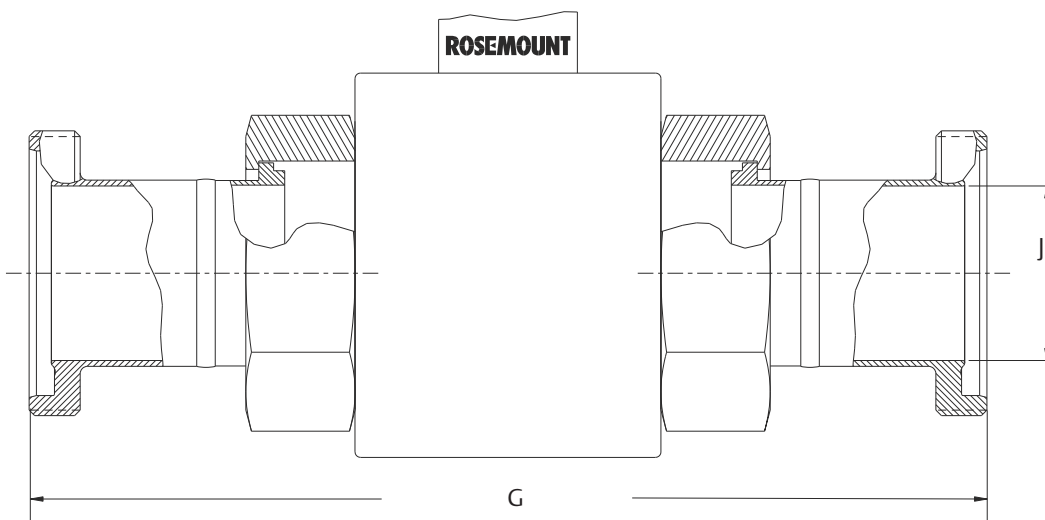
Рисунок 24. Датчик гигиенического (санитарного) исполнения 8721, DIN 11864-1
