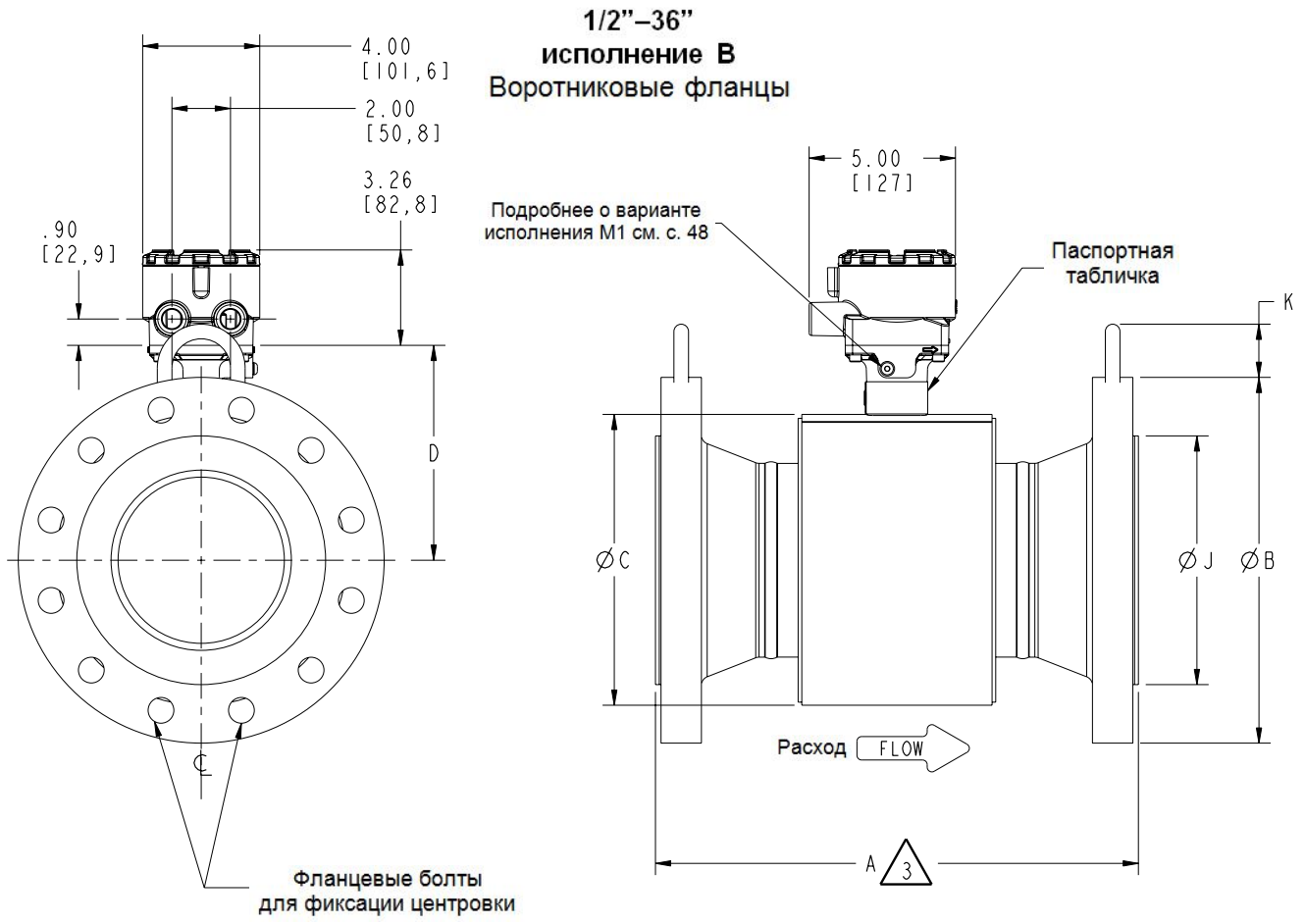
Рисунок 11. Фланцевый датчик 8705-М, типоразмер от 1/2 дюйма до 36 дюймов (DN 15–900 мм), воротниковый фланец, (P ≤ класс 600, сниженные характеристики)
