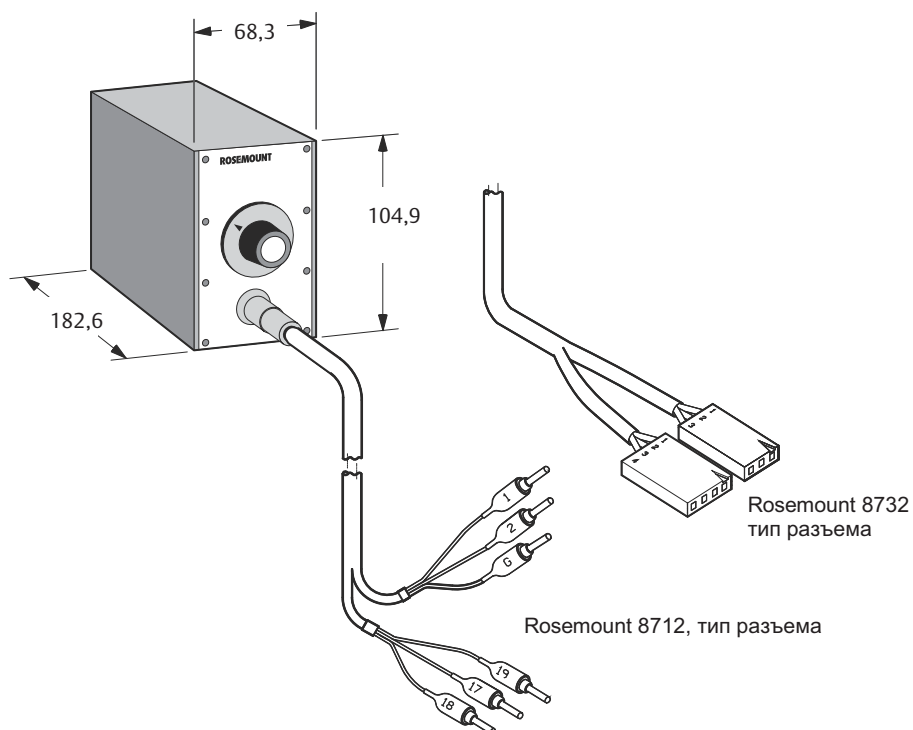
Рисунок 28. Имитатор электромагнитного расходомера Rosemount 8714D — стандартный калибровочный
