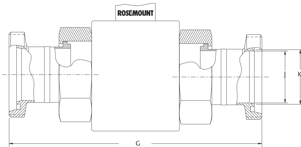
Рисунок 24. Датчик гигиенического (санитарного) исполнения 8721, DIN 11864-1
