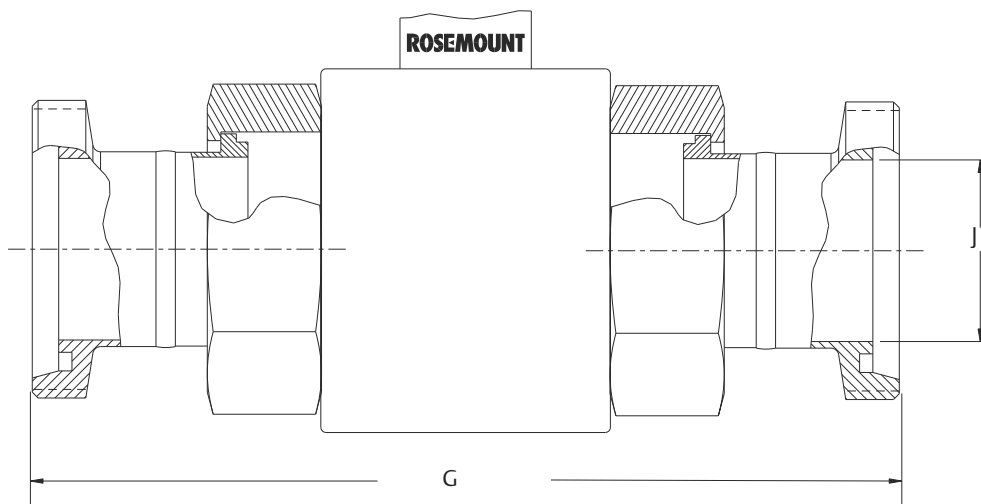
Рисунок 23. Датчик гигиенического исполнения 8721, DIN 11851 (метрическая система)
