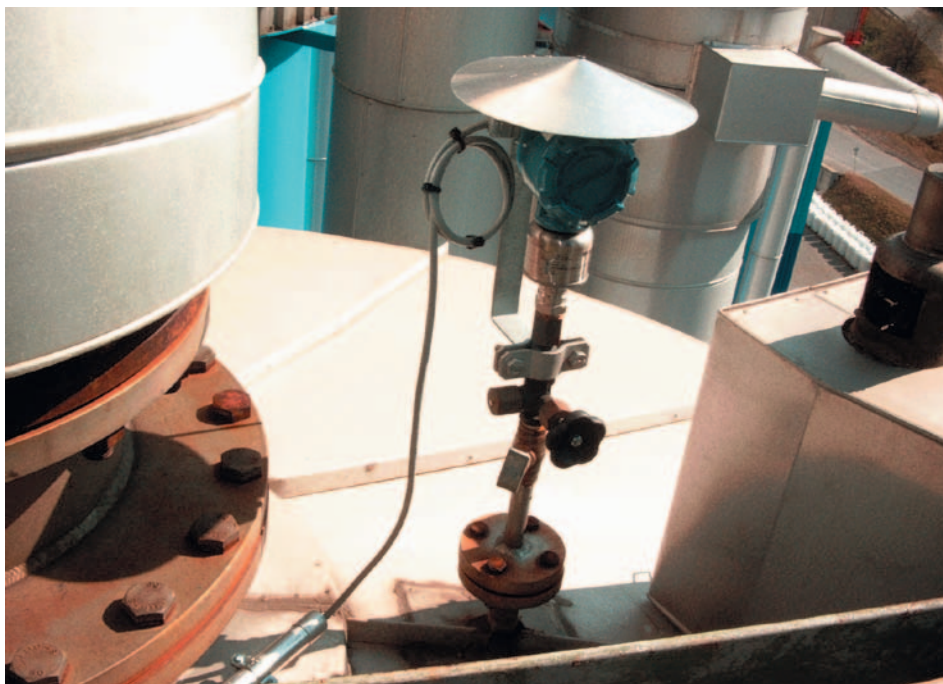
Рис. 3. Сенсор ERS низкого давления, установленный наверху резервуара
