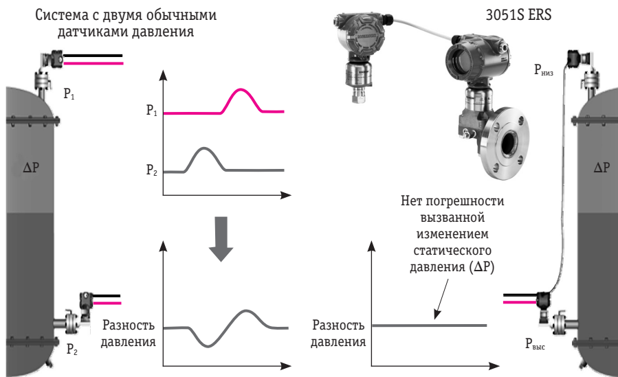
Рис. 1. Установка системы электронных выносных сенсоров Rosemount 3051S ERS
