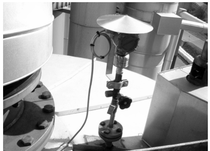
Рис. 3. Сенсор ERS низкого давления, установленный наверху резервуара
