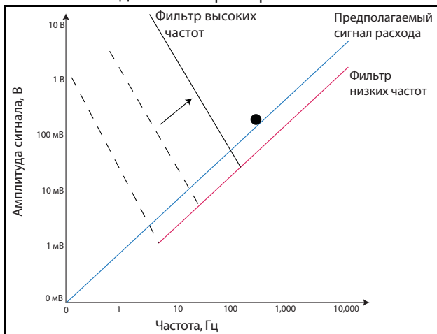
Рис. 7. Адаптивный фильтр высоких частот
