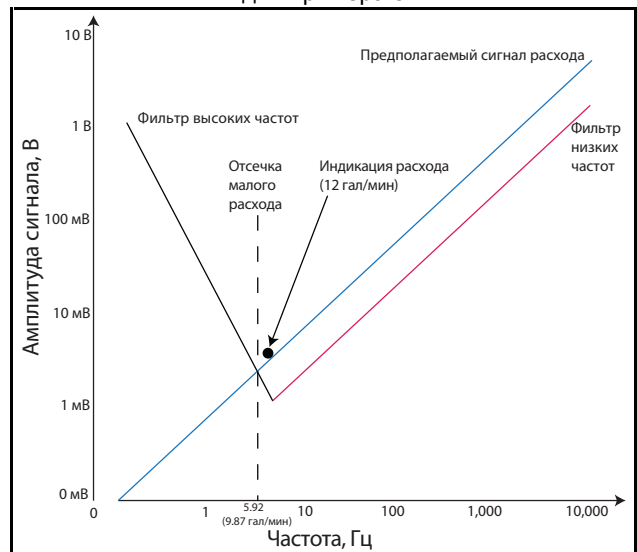
Рис. 25 Настройки фильтра по умолчанию для примера 3
