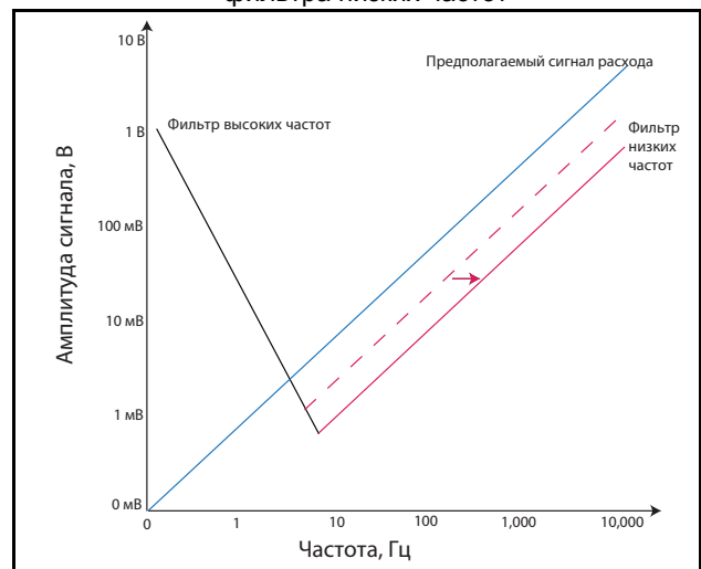
Рис. 19. Регулировка частоты среза фильтра низких частот
