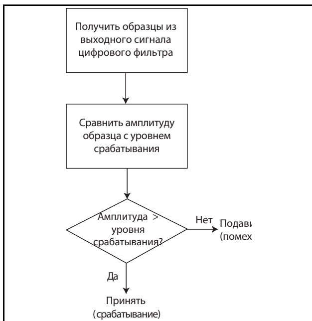
Рис. 9. Блок-схема определения порога (триггер Шмитта)
