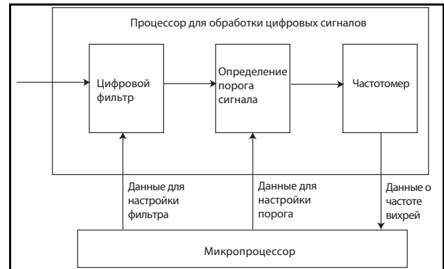
Рис. 8 Движение данных внутри процессора
