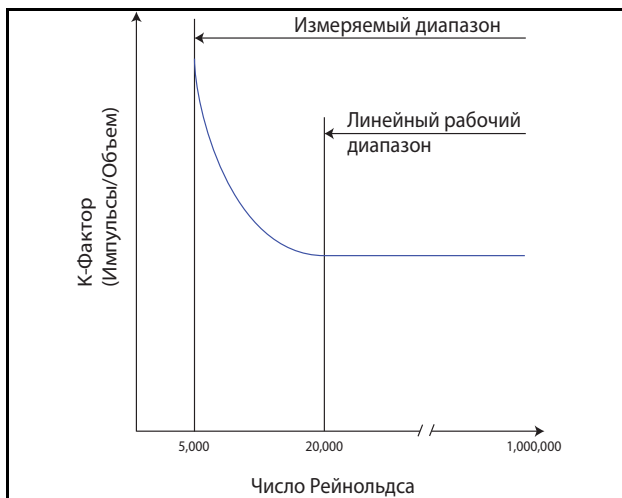
Рис. 1. Зависимость К-фактора от числа Рейнольдса
