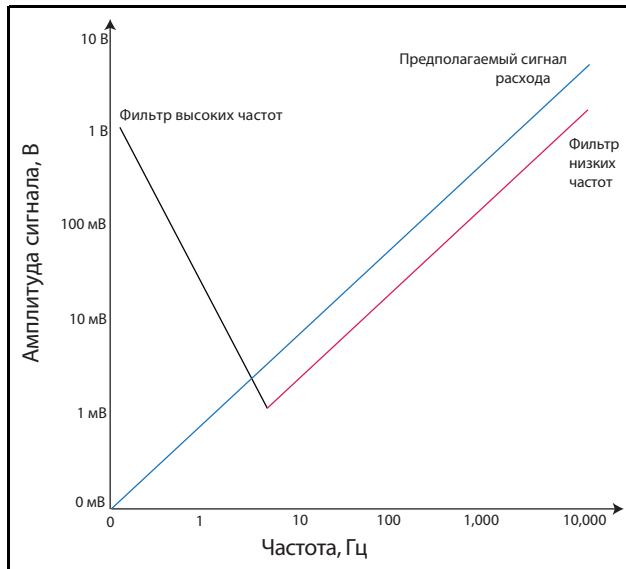
Рис. 4. Диапазон цифровой фильтрации
