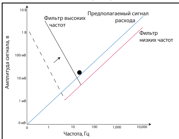
Рис. 6. Адаптивный фильтр высоких частот
