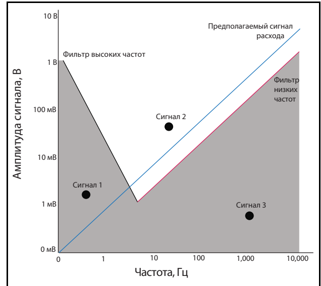
Рис. 5. Измерение сигнала расхода и подавление помех
