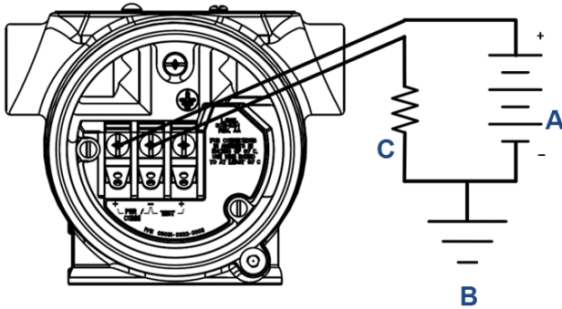
그림 5-1: 트랜스미터 배선도
