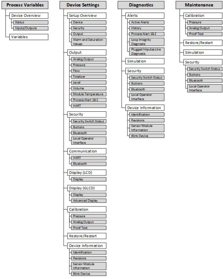
그림 6-1: 장치 드라이버(DD) 메뉴 트리
