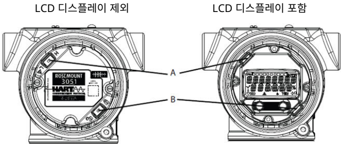
그림 4-1: 전자장치 보드
