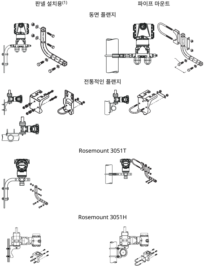
그림 2-1: 판넬 및 파이프 설치용
