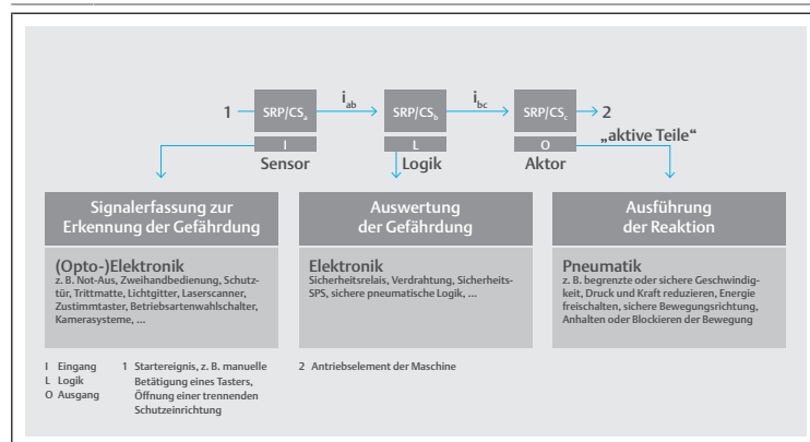
Abb. 2: Fokus auf sicherheitsbezogene Teile einer Steuerung (SRP/CS nach ISO 13849-1)
