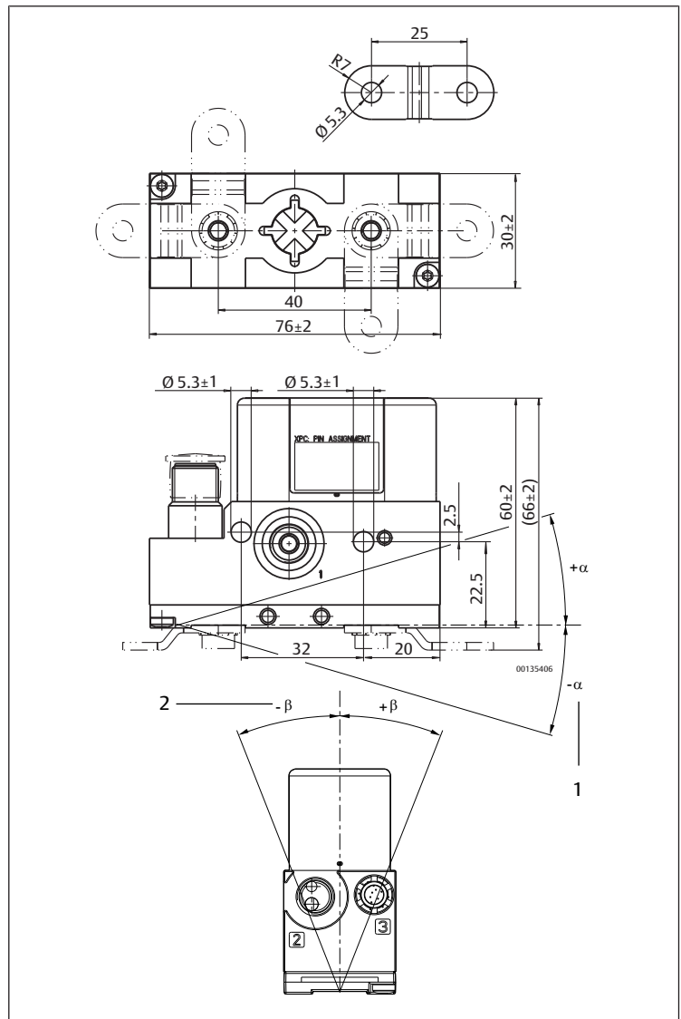
Fig. 6: Plan coté
