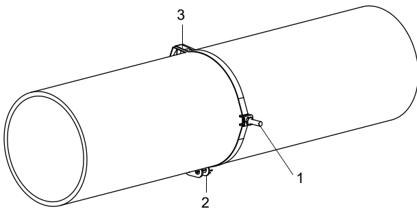
Abb. 6.50: Spannband mit Spannbandklammer und Metallfeder am Rohr
