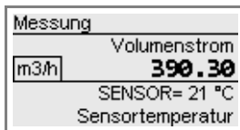
Abb. 9.7: Anzeigen der Sensortemperatur
