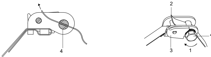
Abb. 6.55: Ratschenschloss mit Spannband
