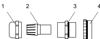
Abb. 7.31: Kabelverschraubung
