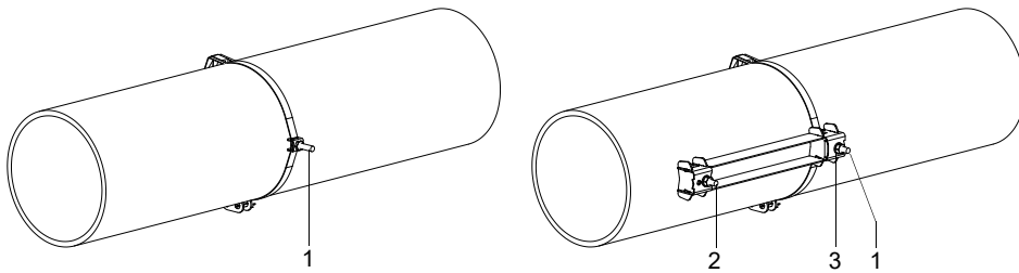
Abb. 6.32: Schiene einseitig am Rohr befestigt
