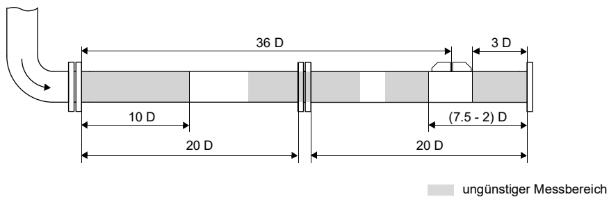
Abb. 3.12: Bereich für die Messstelle mit günstigem Strömungsprofil und geringem Störschalleinfluss
