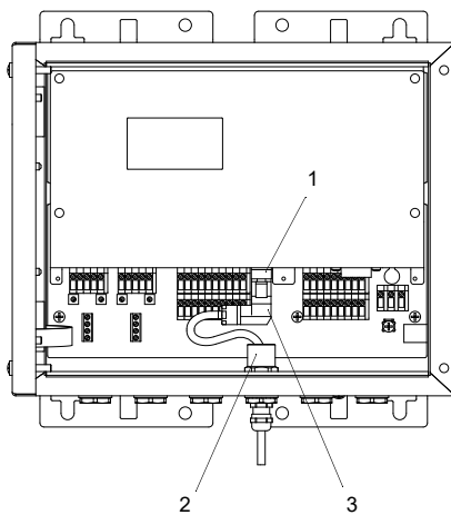
Abb. 7.34: Anschluss des LAN-Kabels
