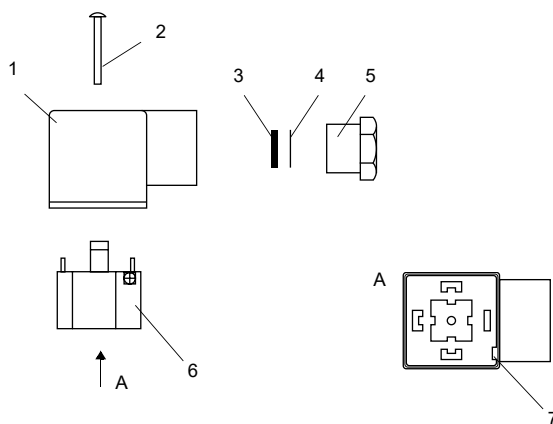
Abb. 7.23: Demontierter Stecker
