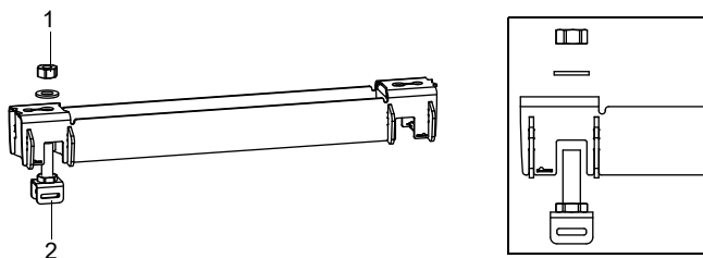
Abb. 6.31: Schiene mit Spannbandklammer
