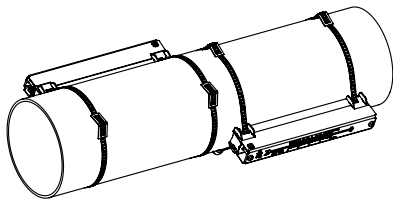
Abb. 6.19: Sensorbefestigung Variofix L (Durchstrahlungsanordnung)
