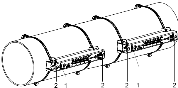
Abb. 6.42: Variofix L mit Sensoren am Rohr
