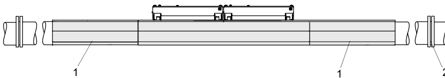
Abb. 6.9: Montierte Sensor- und Rohrdämpfungsmatten in Reflexanordnung
