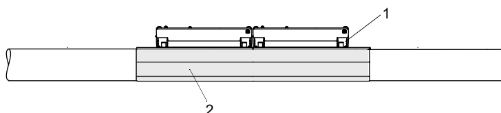
Abb. 6.8: Montierte Sensordämpfungsmatten in Reflexanordnung
