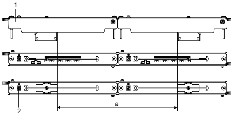
Abb. 6.40: Einstellen des Sensorabstands
