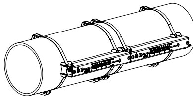
Abb. 6.20: Sensorbefestigung Variofix L (Reflexanordnung)
