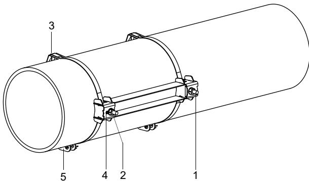
Abb. 6.33: Schiene am Rohr
