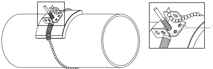
Abb. 6.73: Temperaturfühler am Rohr
