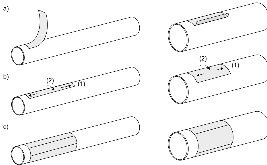
Abb. 6.11: Befestigung der Dämpfungsmatten
