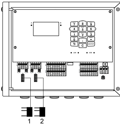
Abb. 7.11: SENSPROM
