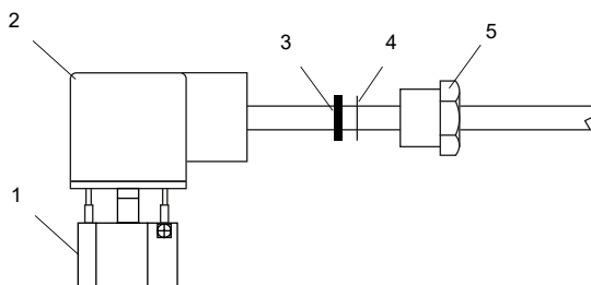
Abb. 7.27: Montage von Stecker und Kabel
