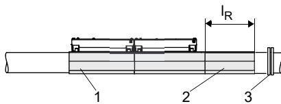
Abb. 6.12: Rohraußendurchmesser < 900 mm
