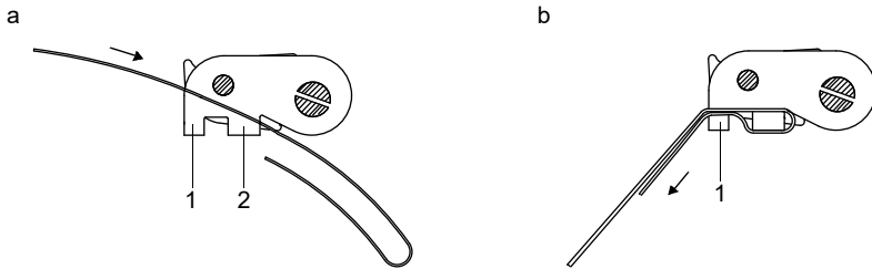
Abb. 6.49: Ratschenschloss mit Spannband
