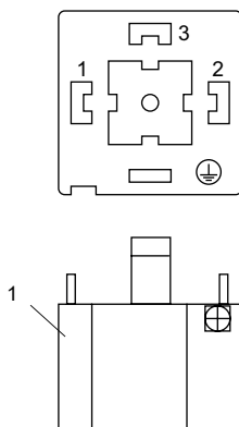
Abb. 7.26: Klemmenbelegung (Stecker)
