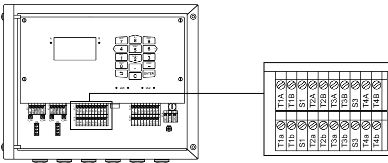
Abb. 7.30: Anschluss der Eingänge am Messumformer
