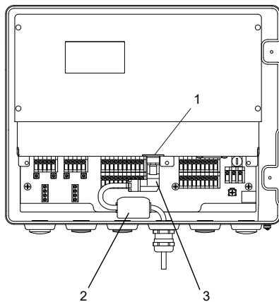
Abb. 7.36: Anschluss des LAN-Kabels
