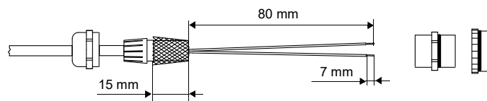
Abb. 7.32: Konfektioniertes Kabel
