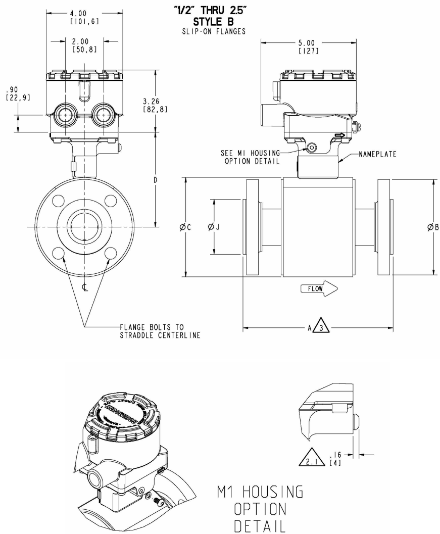
Figura 19: Sensore flangiato 8705-M 1/2" 24" (DN 15 mm - 600 mm) flangia di sovrapposizione - alta pressione (P ≤ Classe 900)
