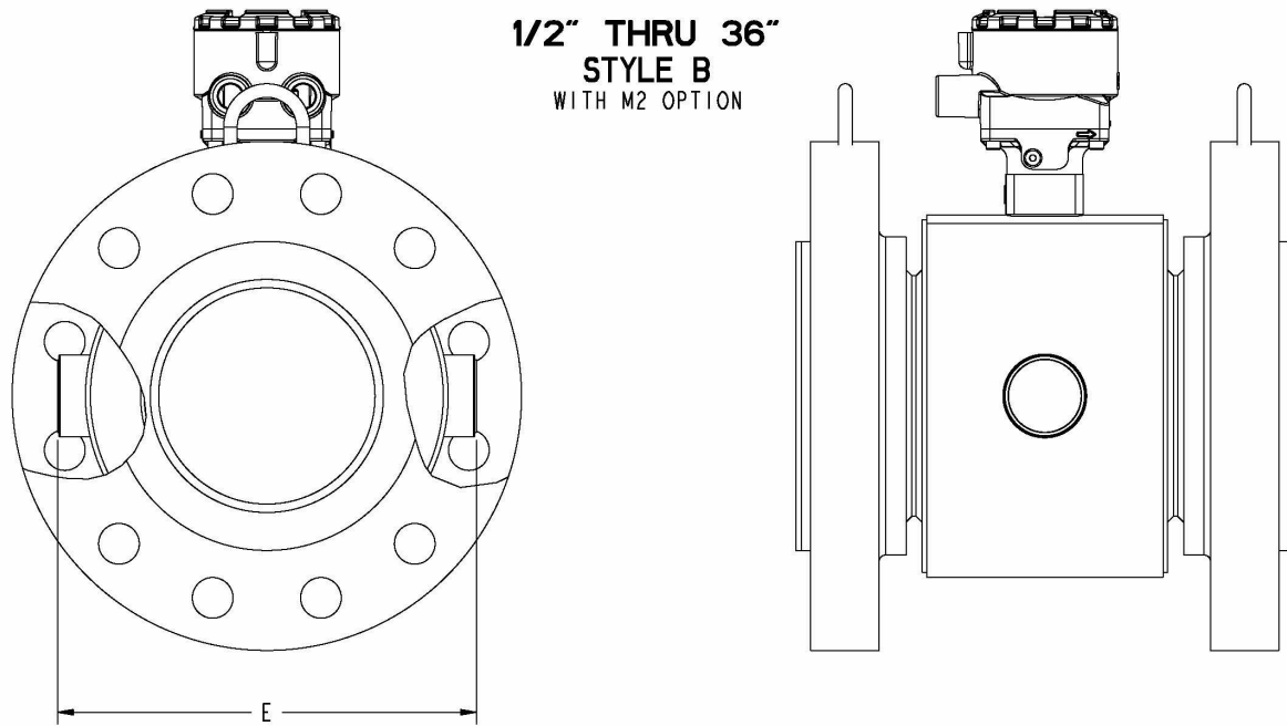
Figura 21: Sensore flangiato 8705-M 1/2" 36" (DN 15 mm - 900 mm) custodia della bobina M2/M4 (P ≤ Classe 2500)
