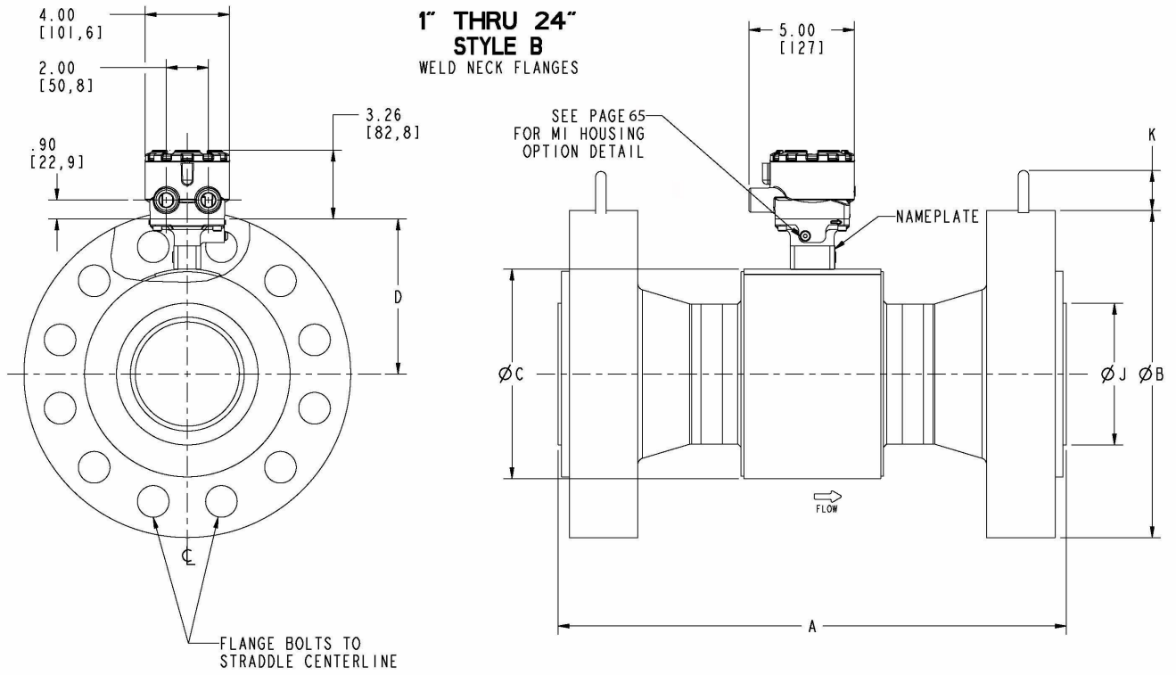
Figura 20: Sensore flangiato 8705-M 1" 24" (DN 25 mm - 600 mm) flangia con colpetto saldato - (P ≤ Classe 2500)
