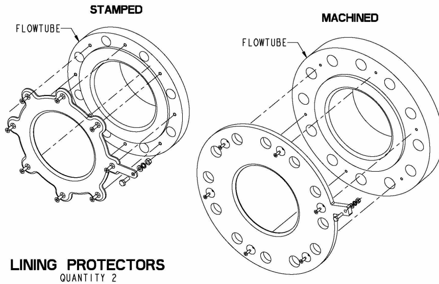
Figura 22: Sensore flangiato 8705-M 1/2" 36" (DN 15 mm - 900 mm) rivestimenti di protezione - (P ≤ Classe 900)
