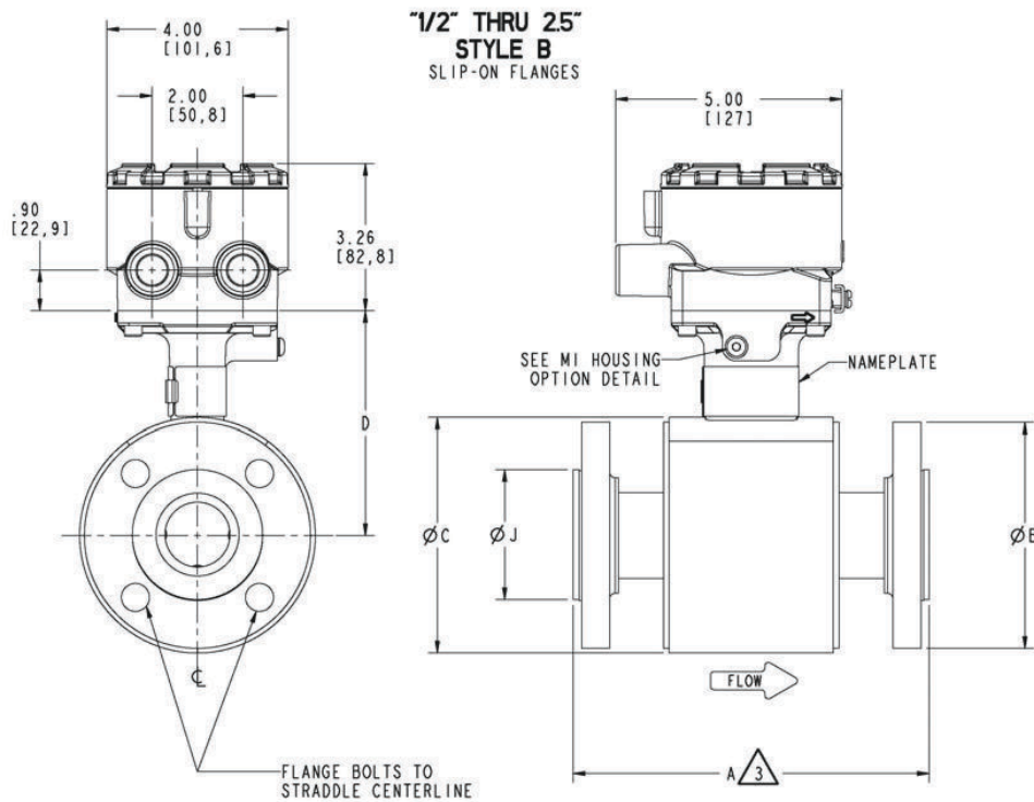
Figura 14: Sensore flangiato 8705-M (DN da 15 mm a 65 mm (da 0,5" a 2,5")) (DN 15 mm to 65 mm) flange a sovrapposizione - bassa pressione (P < Classe 300)
