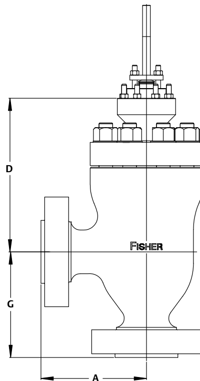
Figur 8. Typiska dimensioner för CL2500 6-steps gjutna NotchFlo DST vinkelventiler (se även tabell 26)
