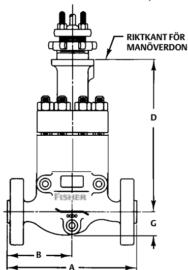
Figur 3. Typiska dimensioner för CL900 och CL1500 v NPS 4, 4-steps NotchFlo DST-sätesventiler (se även tabellerna 16 och 17)
