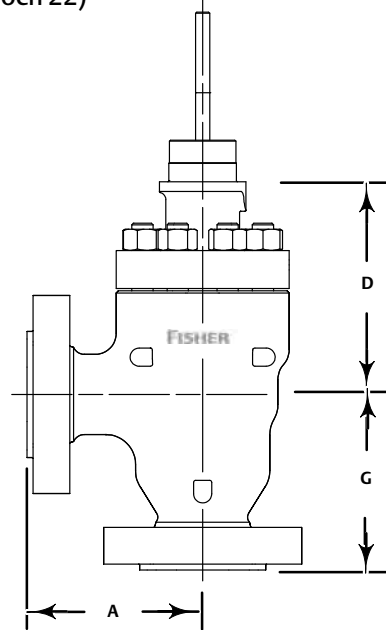
Figur 5. Typiska dimensioner för CL1500 4-steps NotchFlo DST vinkelventil (se även tabell 21 och 22)
