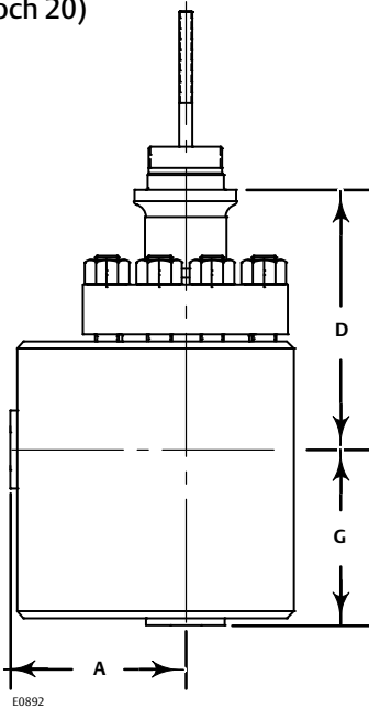
Figur 4. Typiska dimensioner för CL300 3-steps, CL600 3-steps, CL900 4-steps och CL1500 4-steps NotchFlo DST-vinkelventiler (se även tabell 18, 19 och 20)
