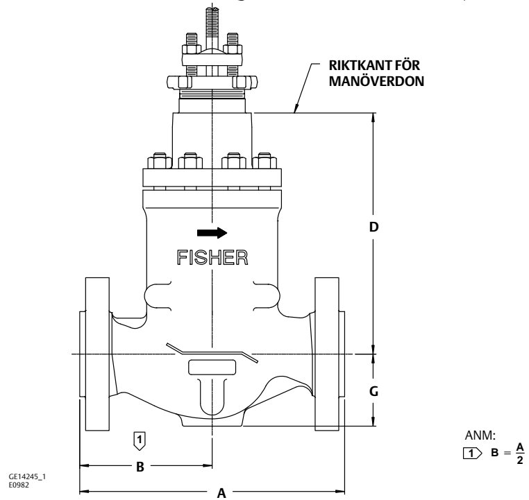
Figur 6. Typiska dimensioner för CL1500 och CL2500 6-stegs NotchFlo DST-kulventiler (se även tabell 23 och 24)
