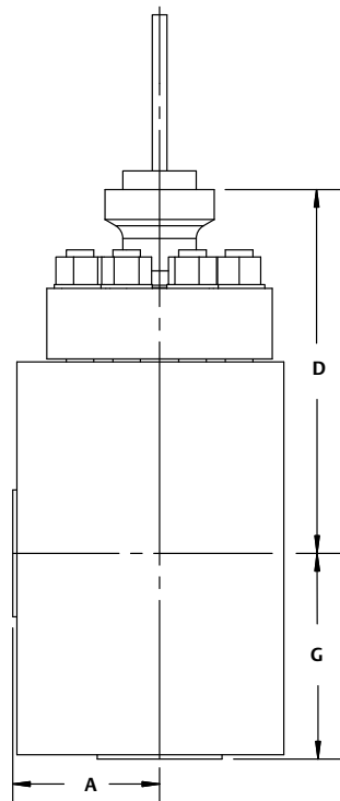
Figur 7. Typiska dimensioner för CL2500 6-steps NotchFlo DST smidda vinkelventiler (se även tabell 25)
