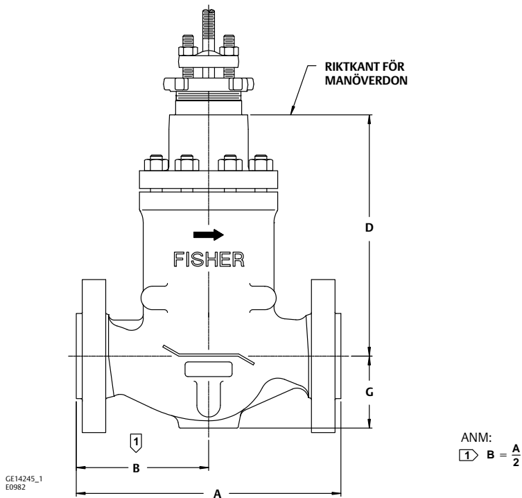
Figur 2. Typiska dimensioner för CL300 och CL600 3-steps NotchFlo DST-ventiler (se även tabell 14 och 15)
