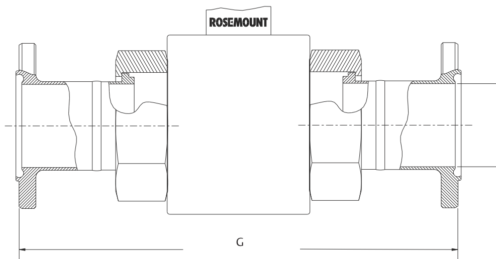
Figura 31: Sensor higiênico (sanitário) 8721 DIN 11864-2
