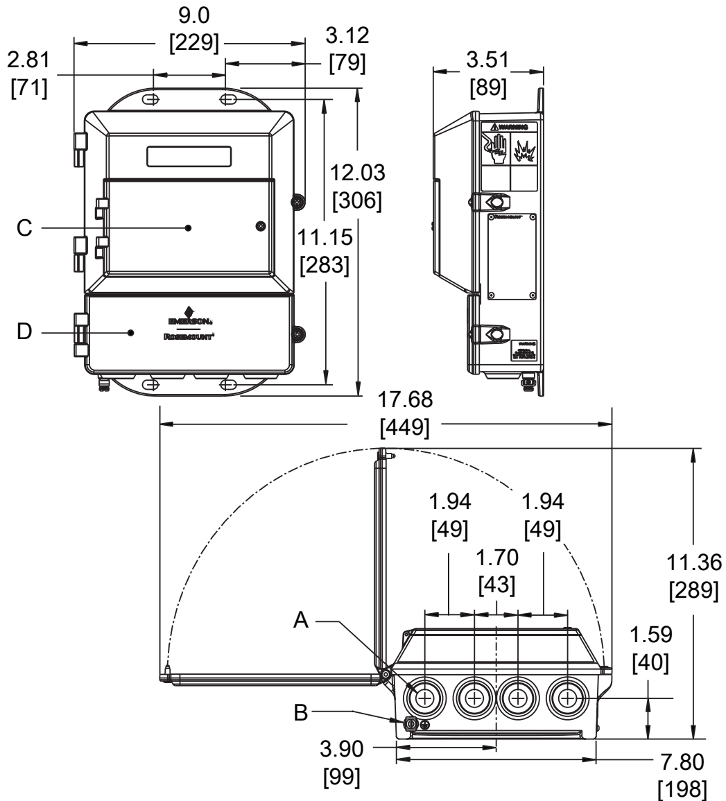
Figura 12: Dimensões do transmissor de montagem na parede 8712
