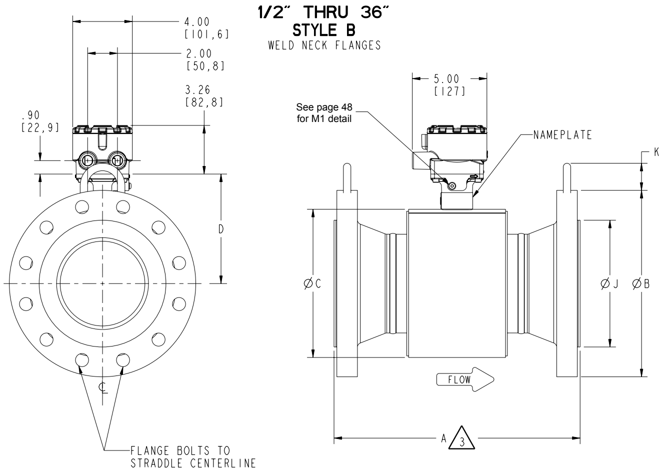
Figura 16: Sensor flangeado 8705-M 1/2 pol. a 36 pol. (DN 15 mm a 900 mm) flanges de pescoço soldado — (P ≤ Classe 600 reduzida)
