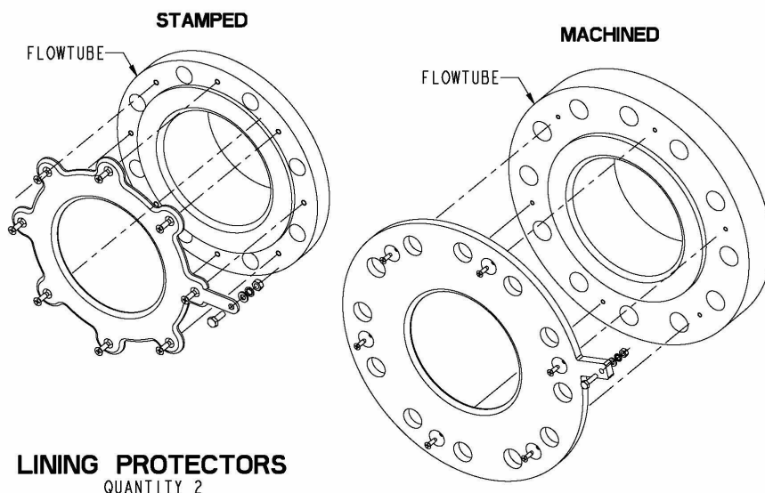
Figura 22: Sensor flangeado 8705-M 1/2 pol. a 36 pol. (DN 15 mm a 900 mm) protetores de revestimento — (P ≤ Classe 900)
