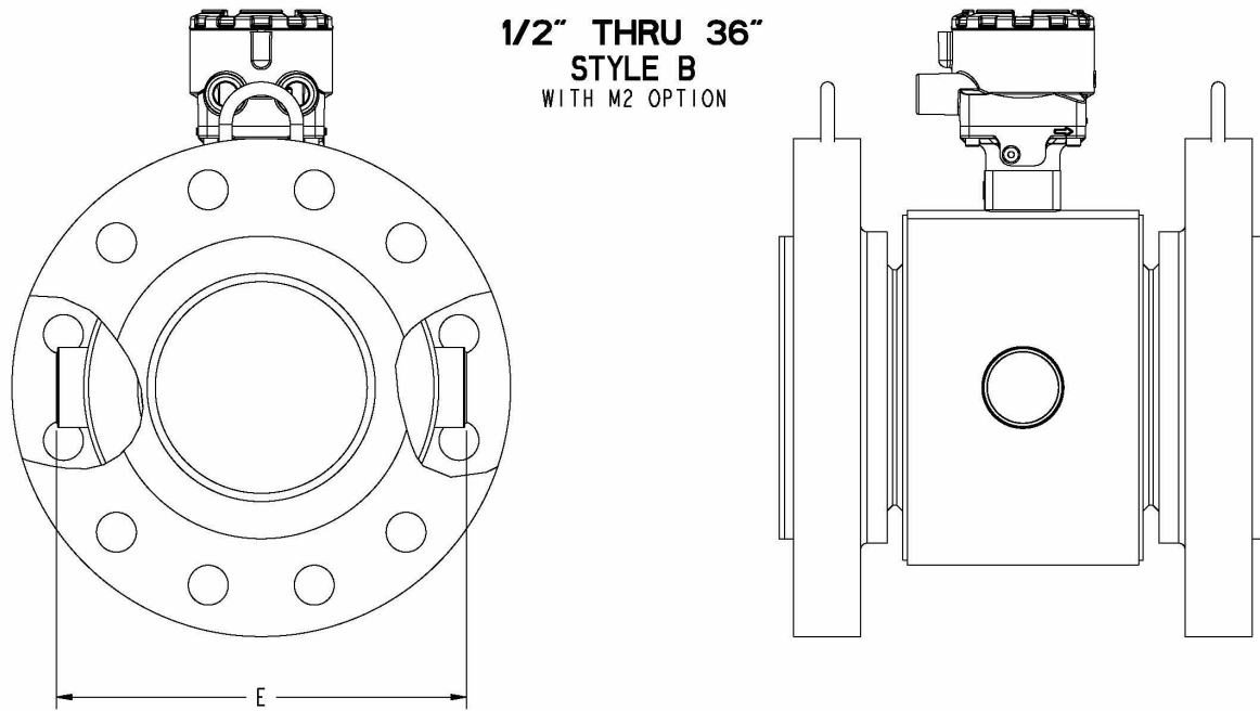
Figura 21: Sensor flangeado 8705-M 1/2 pol. a 36 pol. (DN 15 mm a 900 mm) invólucro da bobina M2/M4 (P ≤ Classe 2500)
