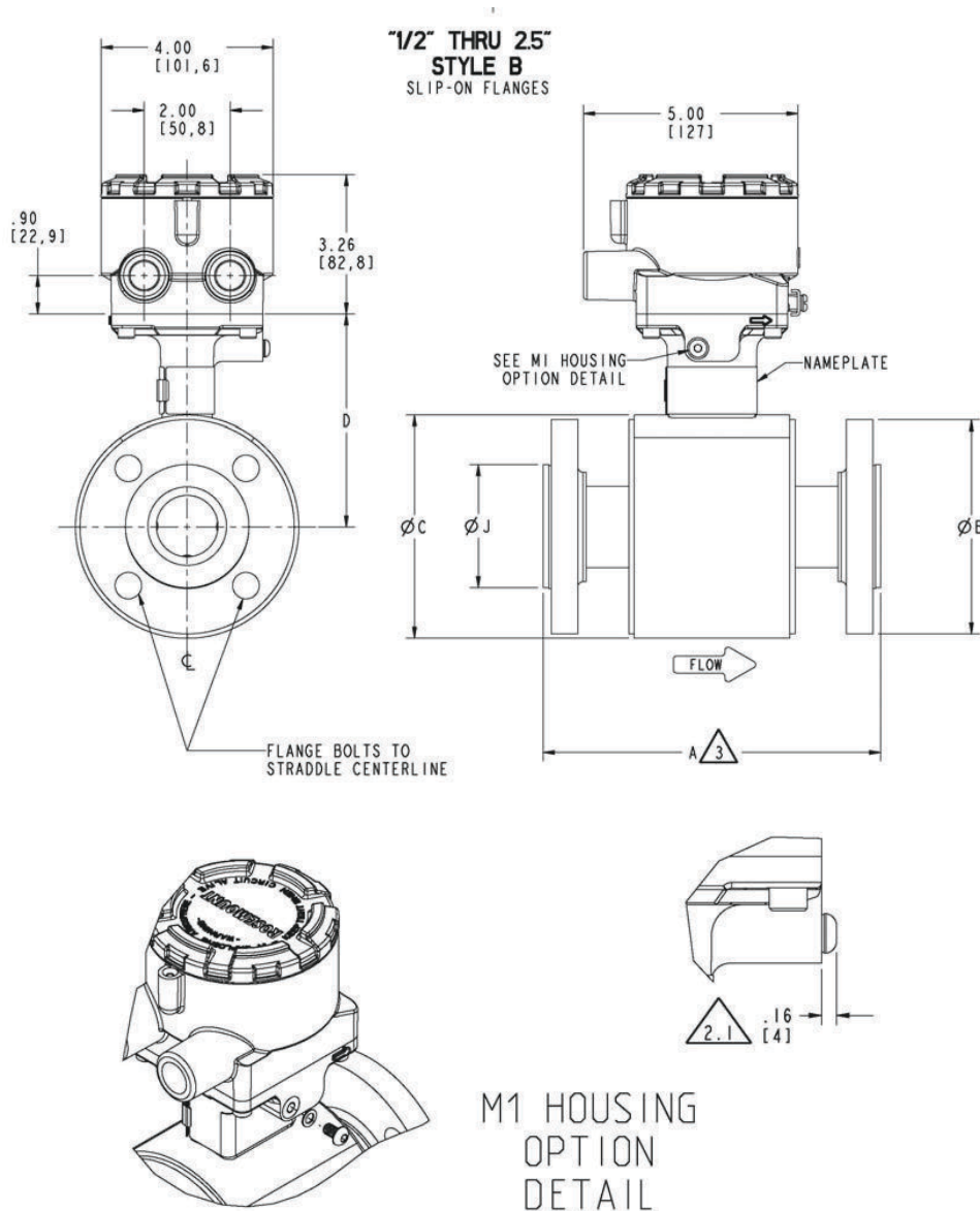
Figura 14: Sensor flangeado 8705-M 0,5 pol. a 2,5 pol. (DN 15 mm a 65 mm) flanges deslizantes — baixa pressão (P < Classe 300)
