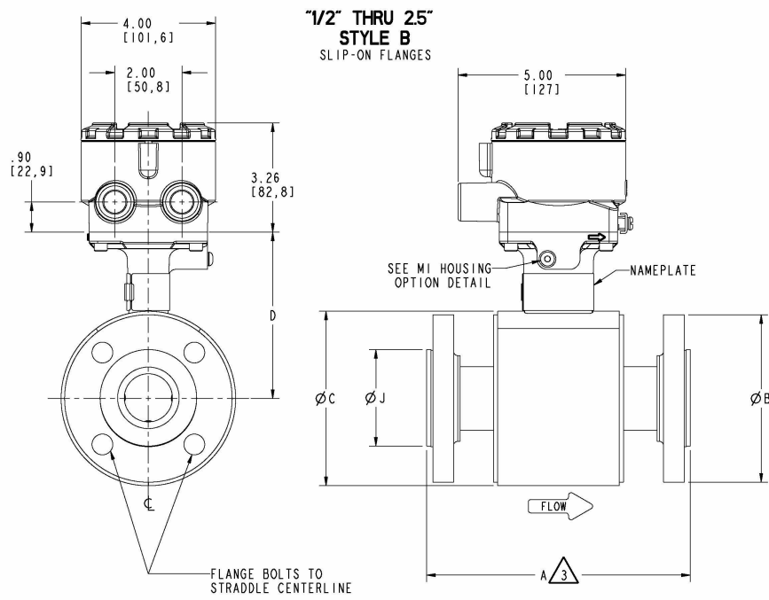
Figura 19: Sensor flangeado 8705-M 1/2 pol. a 24 pol. (DN 15 mm a 600 mm) flange sobreposta - alta pressão (P ≤ Classe 900)
