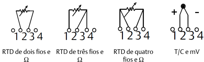
Figura 3-1: Conexões do sensor
