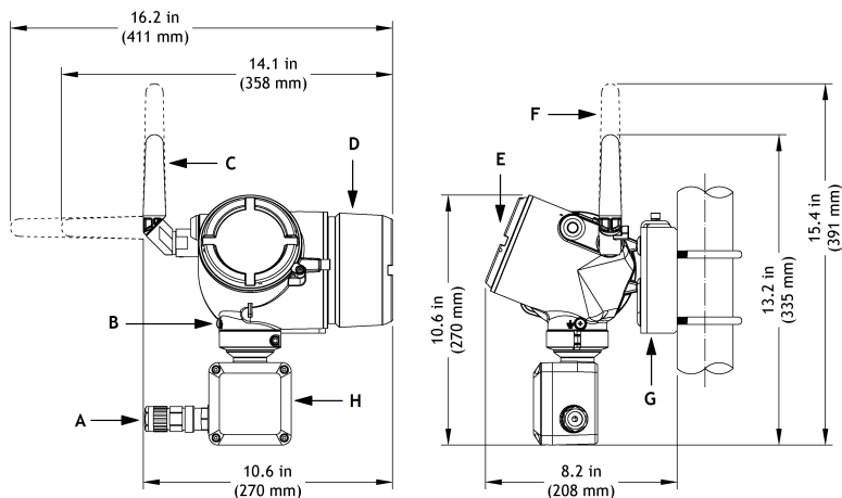
Illustration 6-1 : Dimensions du transmetteur Rosemount 4390
