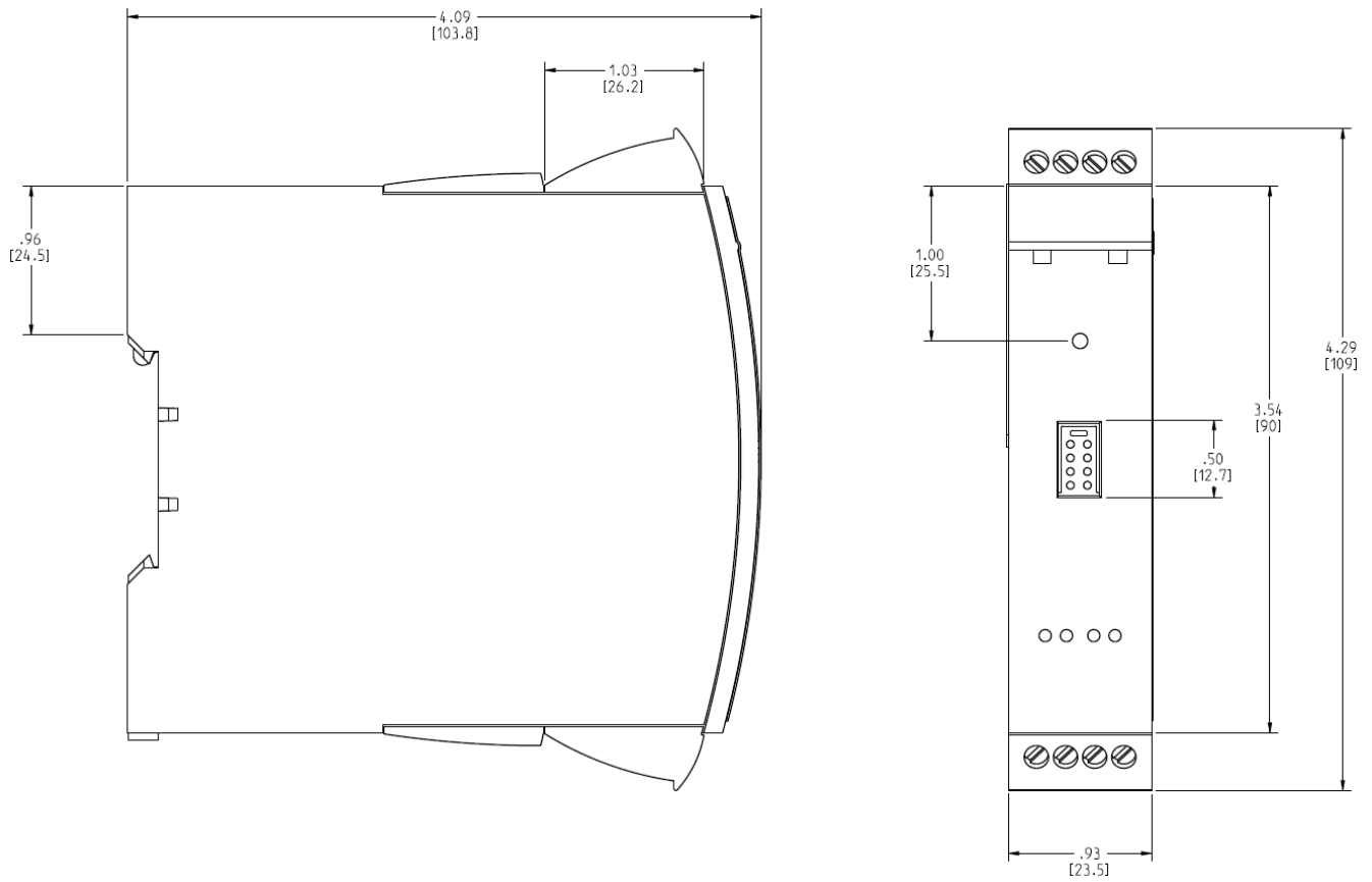
Figura 2: Opción RK del transmisor con montaje en riel Rosemount 248R
