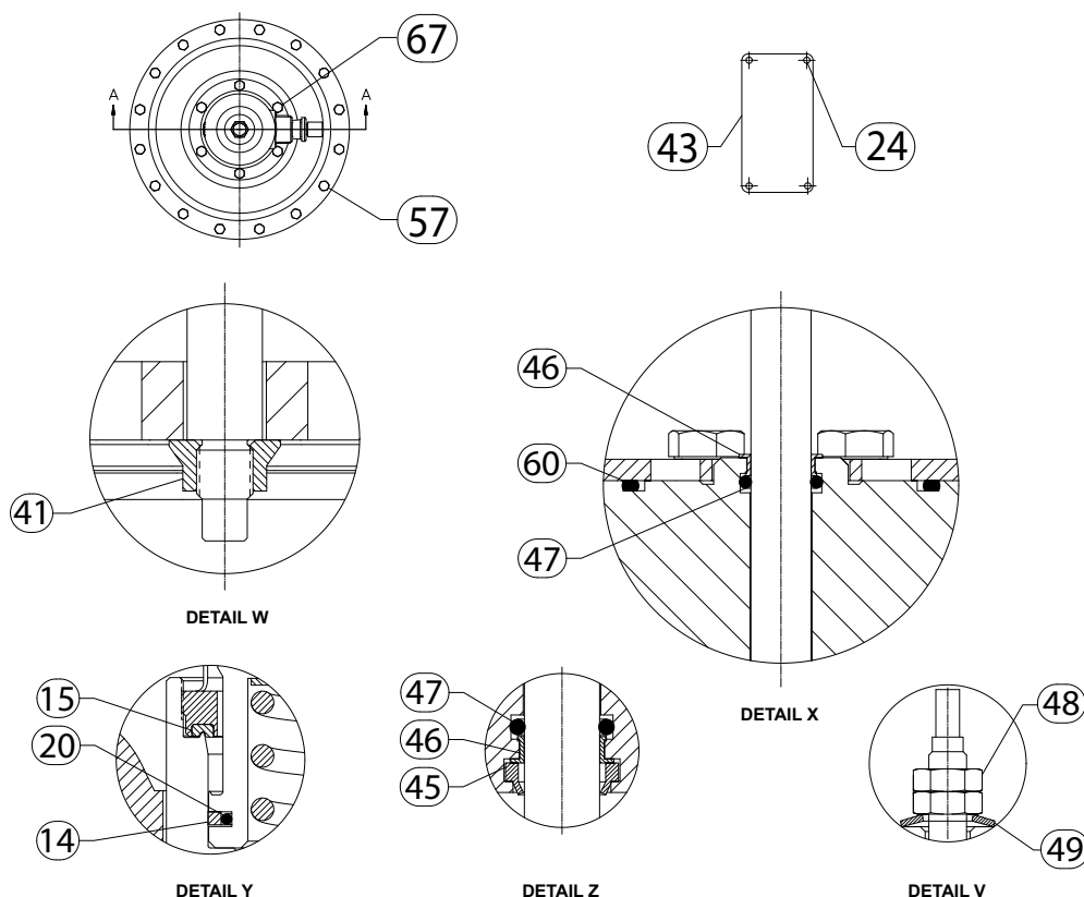
Figure 1. Dessins d'assemblage pour le Type MR108 (suite)
