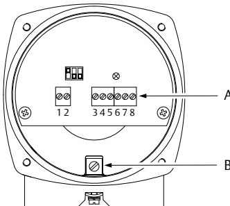
Figur 3-2: PCB-tilslutninger
