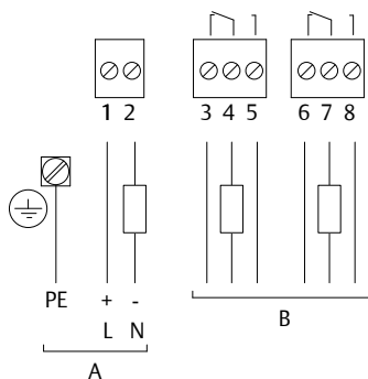
Figur 3-3: Strømforsyning og signaludgang (model med universel spænding)
