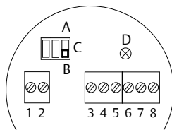
Figur 4-1: FSL- og FSH-indstillinger
