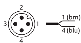
Abb. 1: Anschlussbild Sensor
