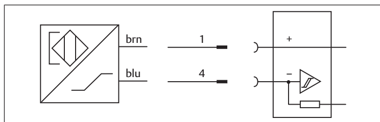
Fig. 1: Schema di collegamento sensore
