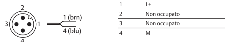
Fig. 1: Schema di collegamento sensore
