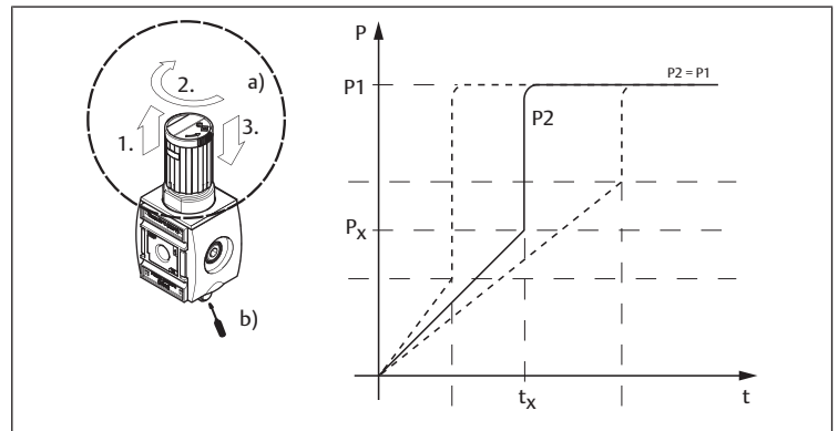
Fig. 10: Válvula de llenado SSV, de accionamiento neumático, tiempo de llenado y presión de conmutación ajustables | Serie AS2, AS3
