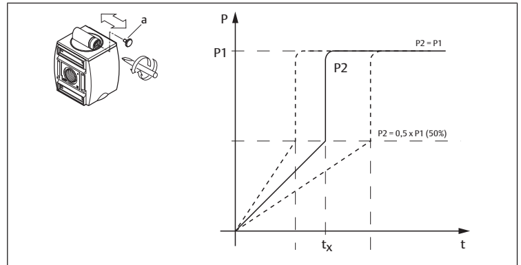
Fig. 9: Válvula de llenado SSV, de accionamiento neumático | Serie AS1, AS2, AS3, AS5
