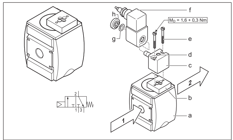
Fig. 8: Válvula distribuidora de 2/2 vías o SOV de 3/2 vías, de accionamiento eléctrico:
