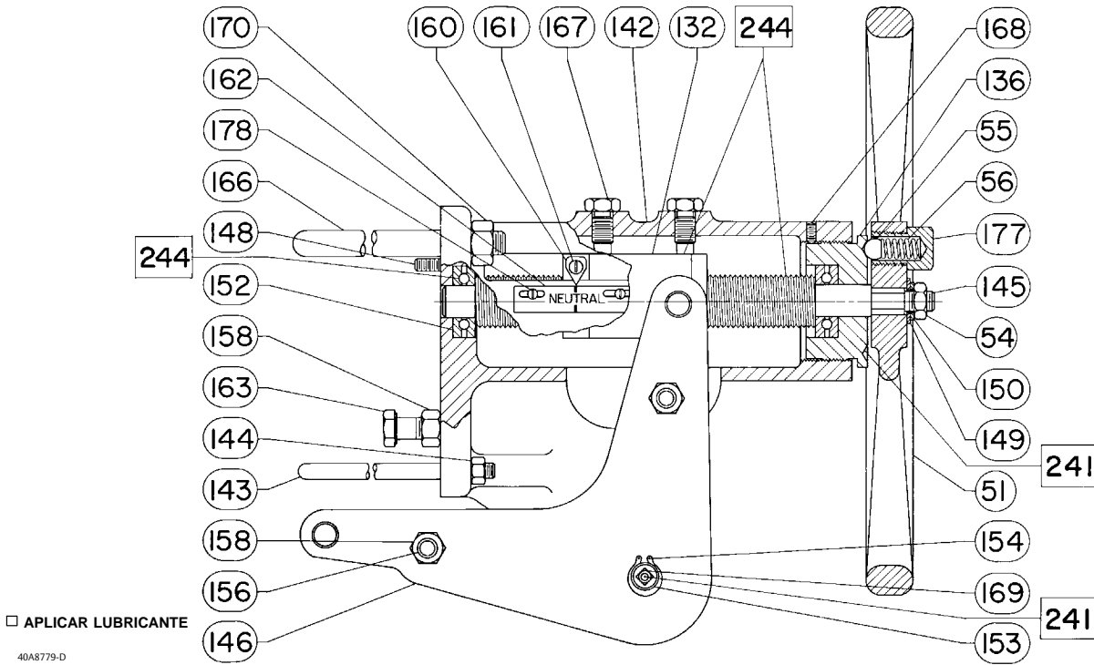
Figura 18. Conjunto de volante de montaje lateral para actuadores de tamaños 45 a 60
