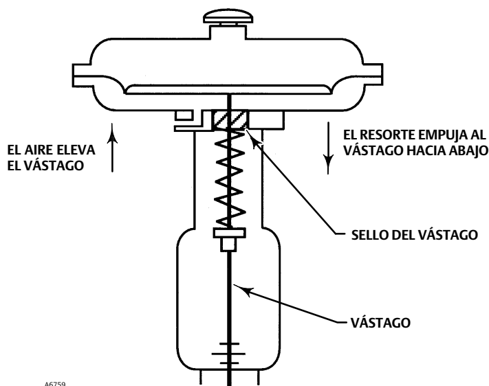
Figura 2. Esquema de los actuadores Fisher 667 y 667-4
