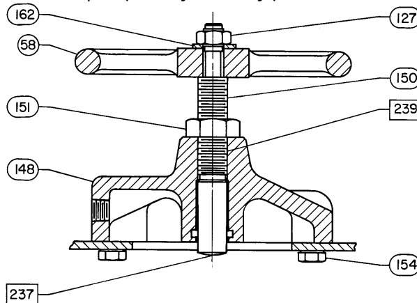
Figura 24. Tope de carrera ascendente estilo 13 - Para tamaños 30/30i a 60/60i y 76/76i se muestra el tamaño 30/30i (montaje en la caja)
