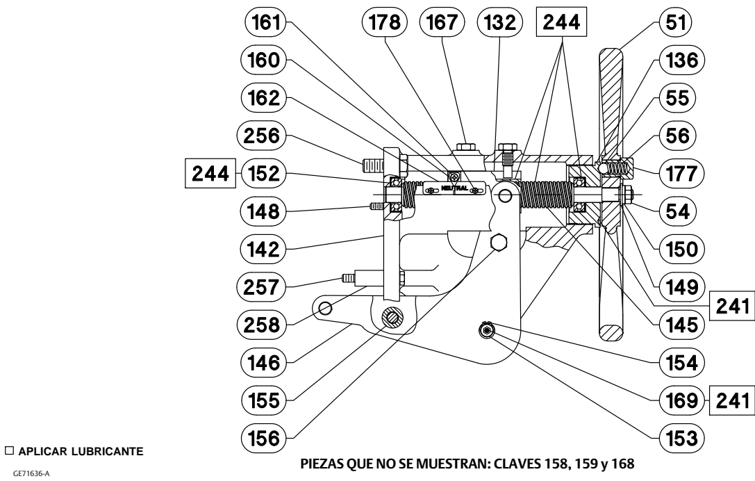
Figura 19. Conjunto de volante de montaje lateral para actuadores de tamaños 45i a 60i
