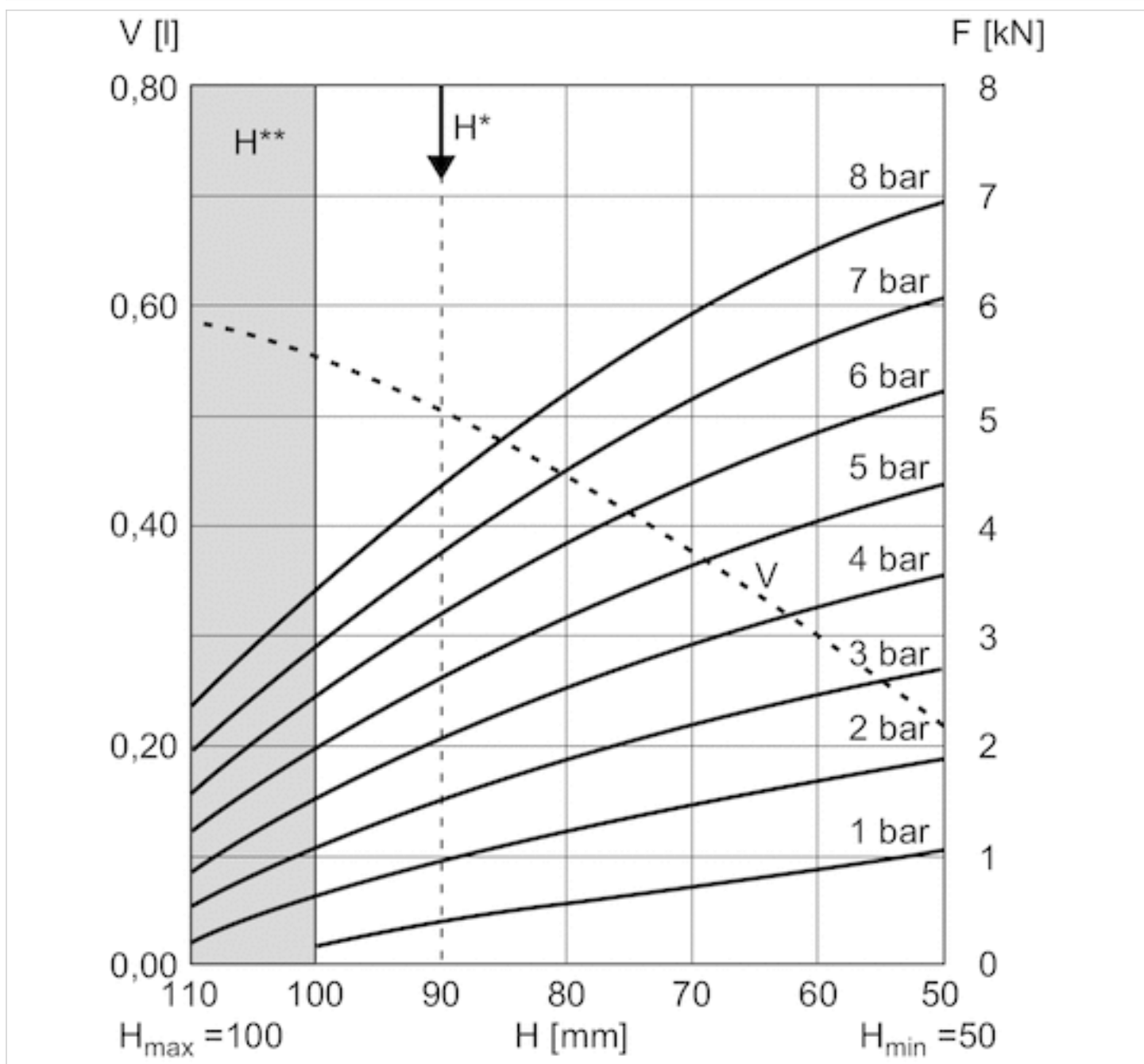
Kraft-Weg-Diagramm, 0822419001
