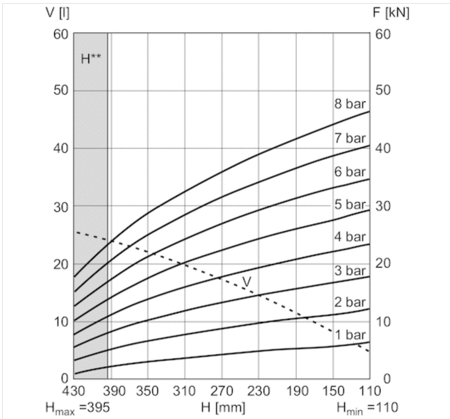
Kraft-Weg-Diagramm, 2999612800
