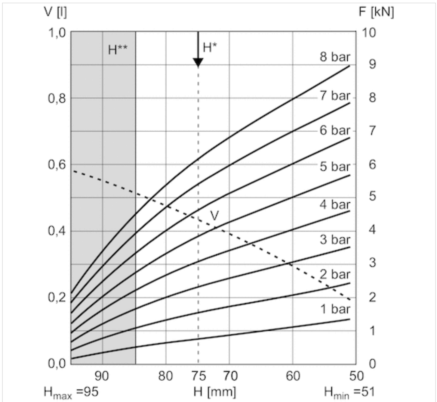
Kraft-Weg-Diagramm, R412010215
