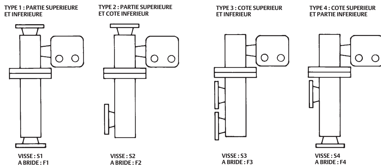
Figure 5. Types de connexion de la cage
