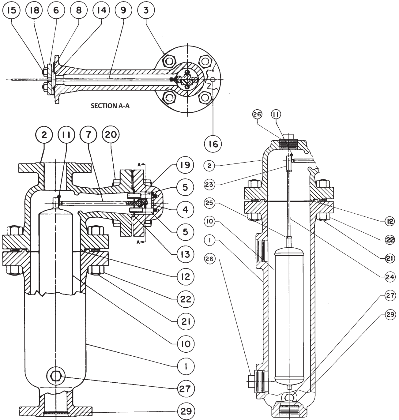
Figure 8. Construction du capteur Fisher 249
