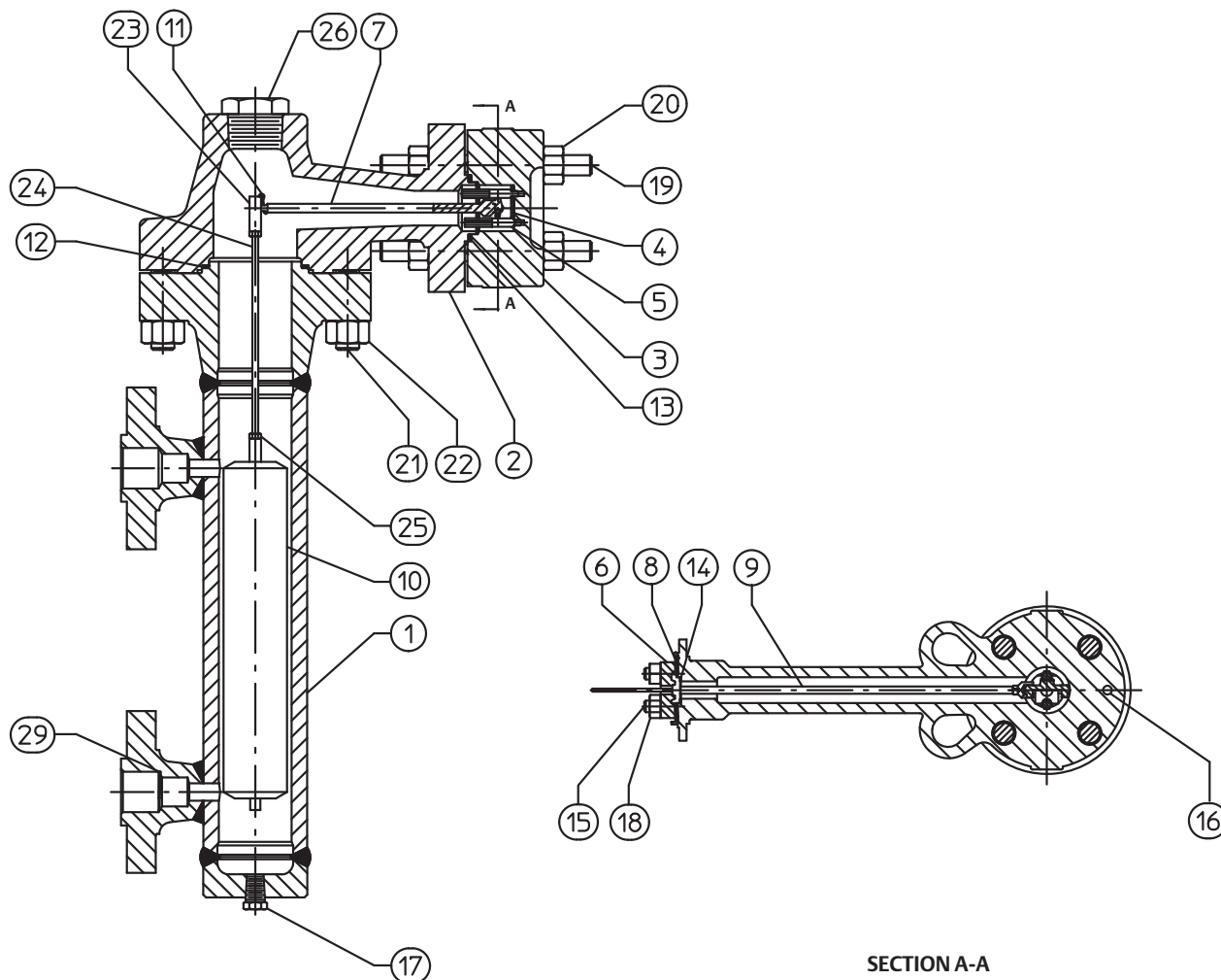
Figure 11. Construction du capteur Fisher 249K
