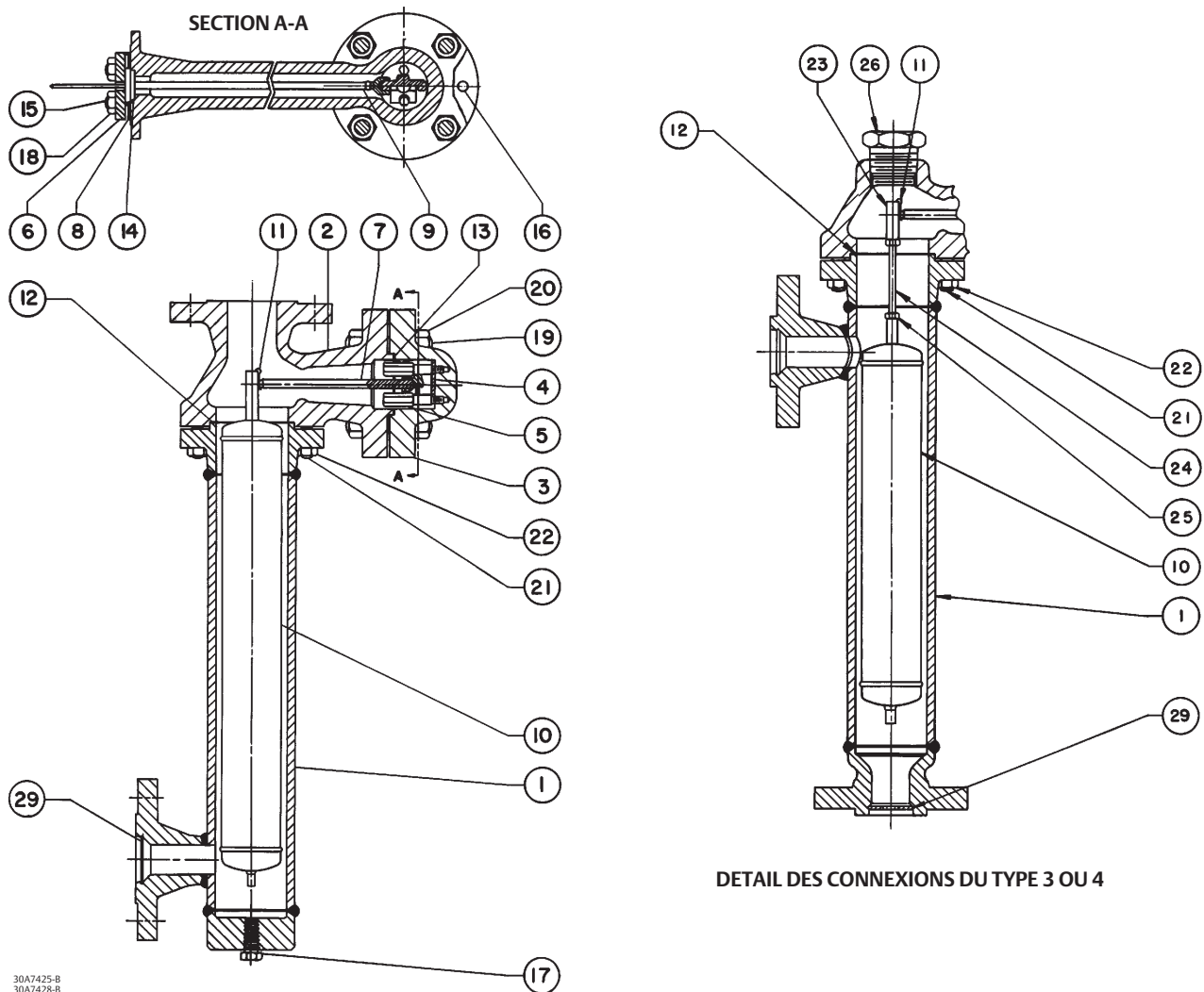
Figure 10. Construction du capteur Fisher 249C
