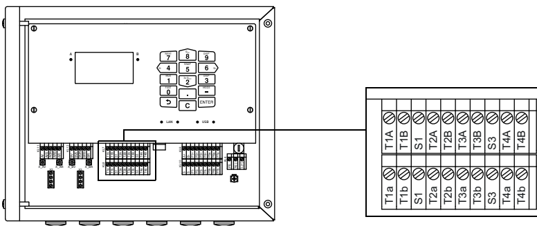
Fig. 7.30: Conexión de las entradas al transmisor
