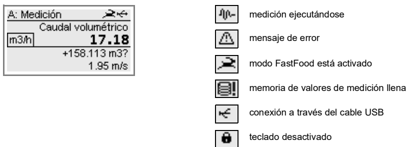
Fig. 4.4: Visualización del estado (línea 1)
