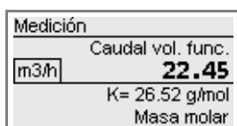
Fig. 9.2: Visualización de los valores de medición
