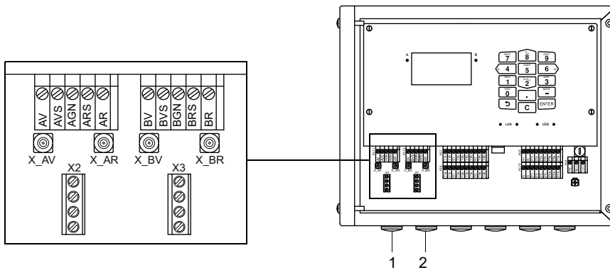
Fig. 7.1: Conexión de los transductores al transmisor
