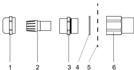
Fig. 7.14: Prensaestopas para carcasa de acero inoxidable
