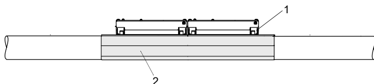
Fig. 6.8: Esteras de amortiguamiento montadas en configuración en modo de reflexión
