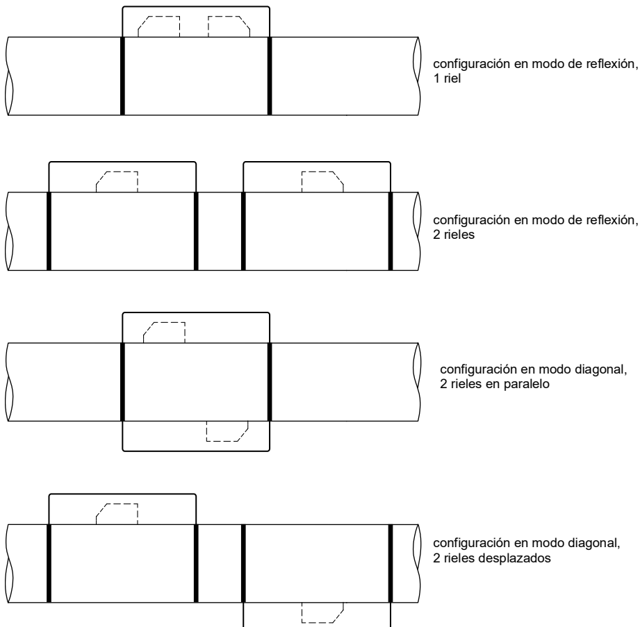
Fig. 6.15: Configuración de los transductores en rieles de montaje
