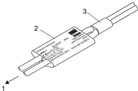
Fig. 6.18: Placa de características en el cable del transductor
