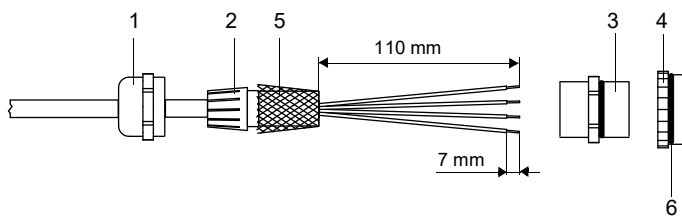
Fig. 7.19: Confección del sensor de temperatura
