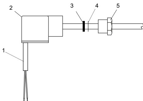
Fig. 7.24: Montaje del cable
