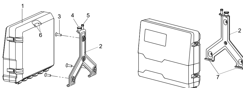
Fig. 6.5: Vista de montaje
