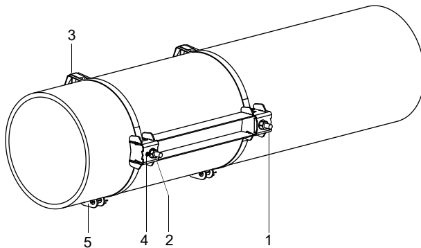
Fig. 6.33: Riel en la tubería
