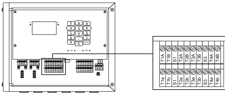
Fig. 7.17: Conexión de las entradas al transmisor
