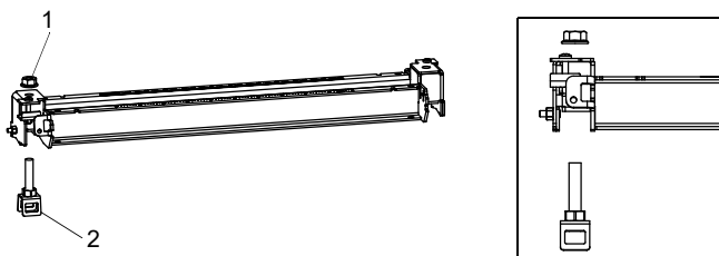
Fig. 6.56: Riel con sujetador para cinta de sujeción
