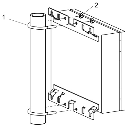
Fig. 6.6: Vista de montaje
