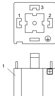
Fig. 7.26: Conexión de bornes (conector)
