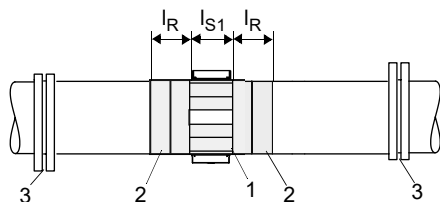
Fig. 6.13: Diámetro exterior de la tubería > 900 mm
