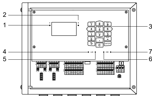
Fig. 8.1: Panel de mando del transmisor
