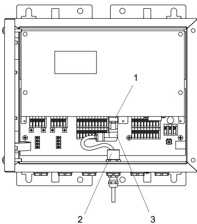
Fig. 7.34: Conexión del cable LAN
