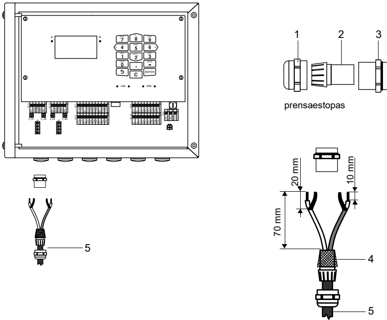
Fig. 7.5: Conexión de la extensión en el transmisor
