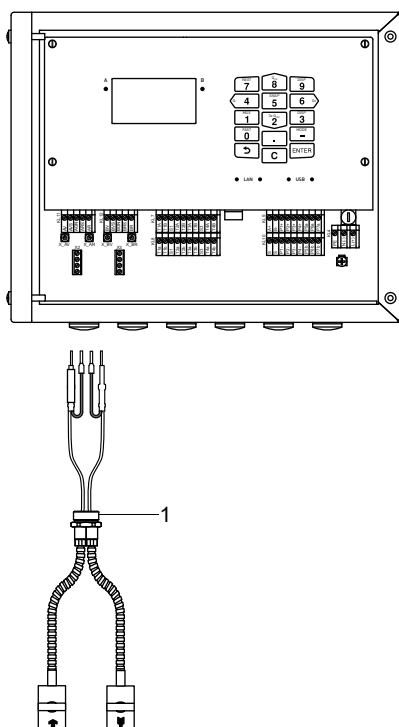
Fig. 7.4: Conexión del cable del transductor con revestimiento de acero inoxidable y extremos pelados al transmisor
