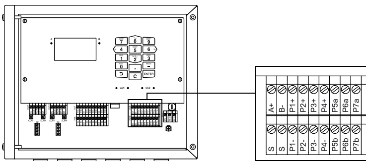
Fig. 7.16: Conexión de salidas al transmisor
