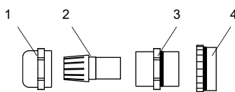
Fig. 7.31: Prensaestopas
