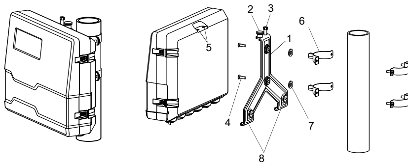
Fig. 6.7: Vista de montaje
