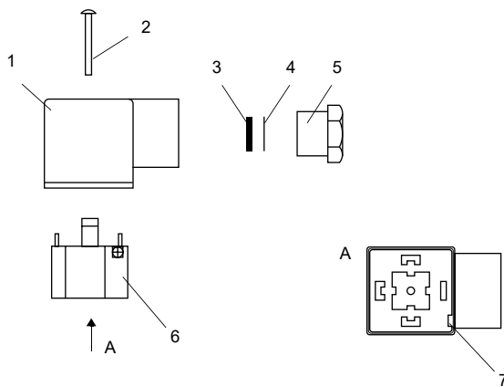
Fig. 7.23: Conector desmontado
