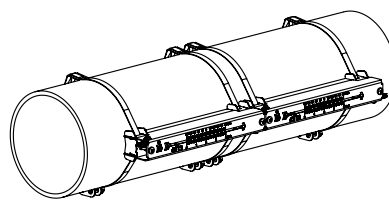
Fig. 6.20: Porta-transductor Variofix L (configuración en modo de reflexión)
