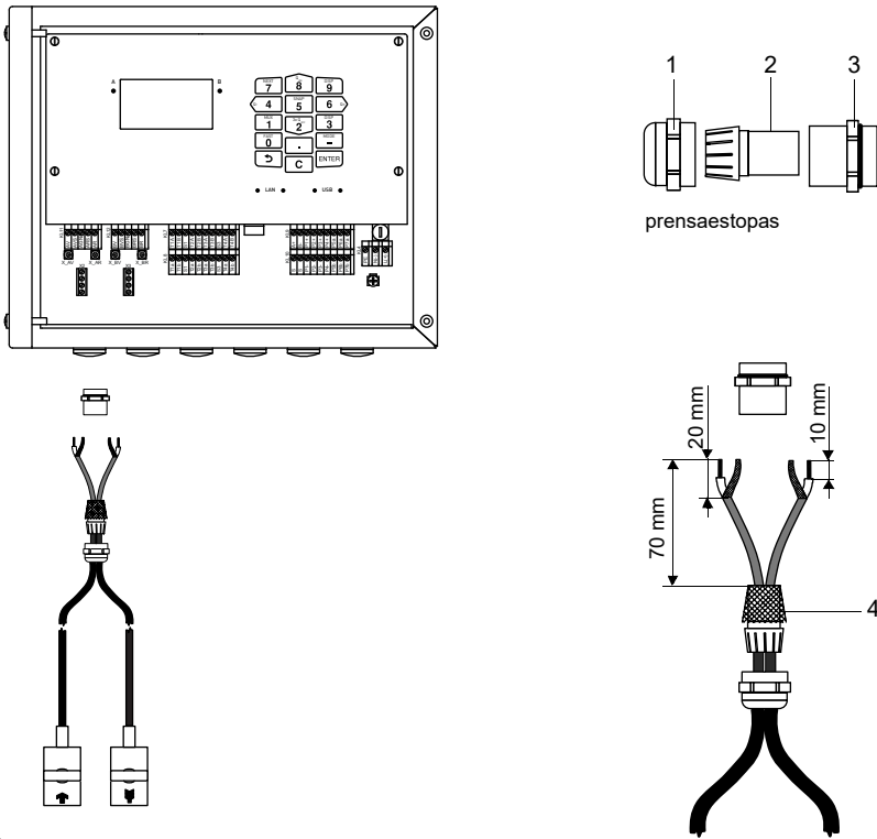
Fig. 7.3: Conexión del cable del transductor con cubierta exterior de plástico y extremos pelados al transmisor
