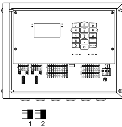
Fig. 7.11: Memoria SENSPROM
