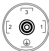
Fig. 7.29: Contactos machos del transmisor de presión
