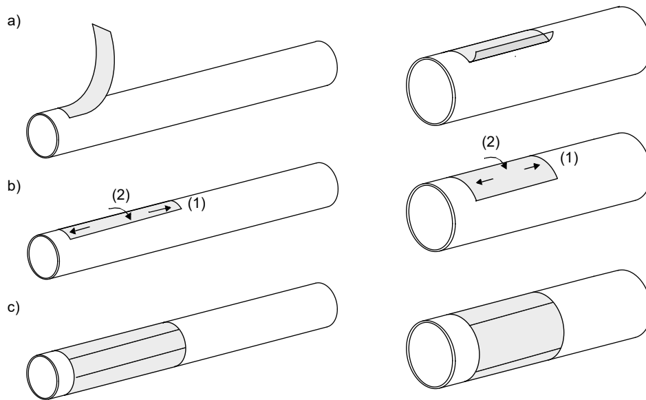
Fig. 6.11: Fijación de la esteras de amortiguamiento
