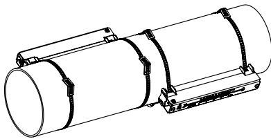
Fig. 6.19: Porta-transductor Variofix L (configuración en modo diagonal)
