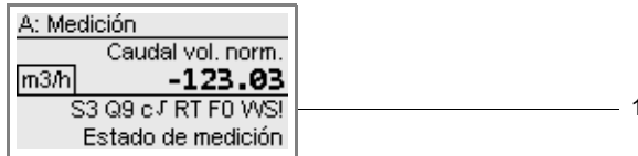
Fig. 9.5: Visualización de la línea de estado
