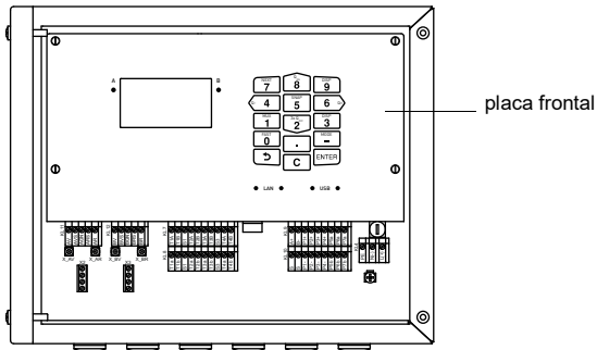
Fig. 2.1: Transmisor
