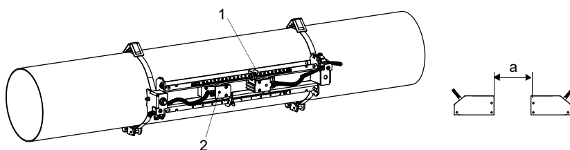
Fig. 6.63: Transductores en el riel (aquí sin estribos elásticos)
