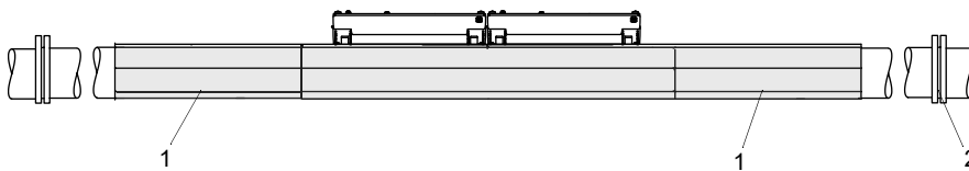
Fig. 6.9: Esteras de amortiguamiento para el transductor y la tubería en configuración en modo de reflexión
