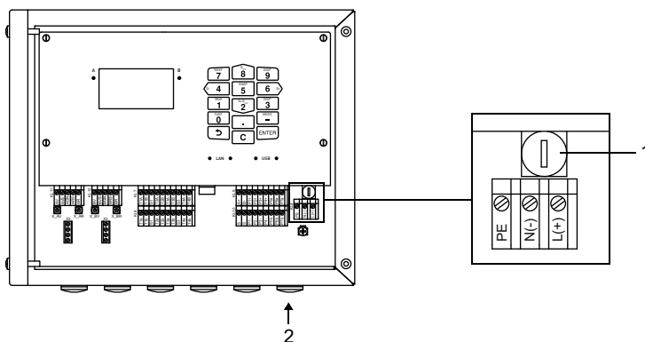
Fig. 7.13: Conexión de la fuente de alimentación al transmisor
