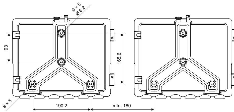
Fig. 6.4: Transmisor (dimensiones en mm)
