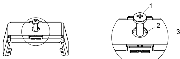
Fig. 6.64: Estribo elástico
