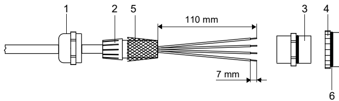
Fig. 7.21: Confección de la extensión
