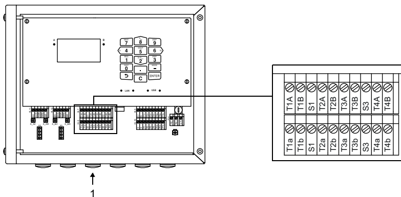
Fig. 7.18: Conexión del sensor de temperatura en el transmisor
