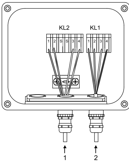
Fig. 7.22: Caja de bornes
