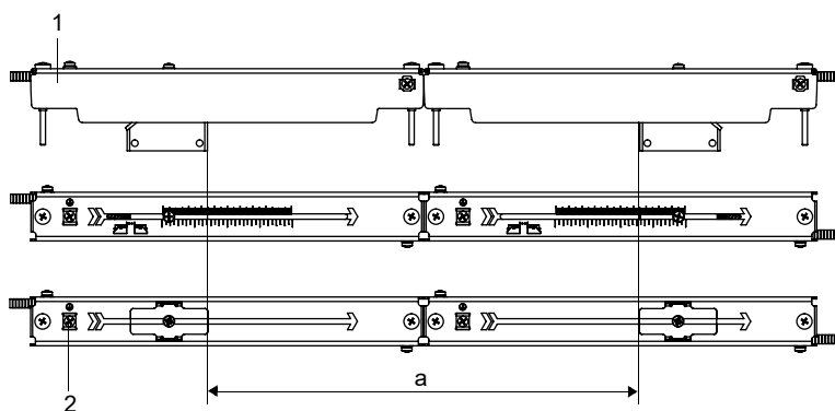
Fig. 6.40: Ajuste de la distancia entre transductores
