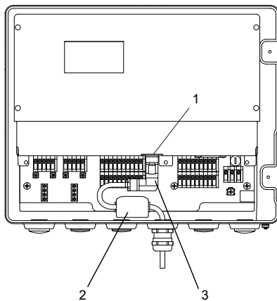
Fig. 7.36: Conexión del cable LAN
