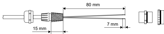
Fig. 7.32: Cable confeccionado
