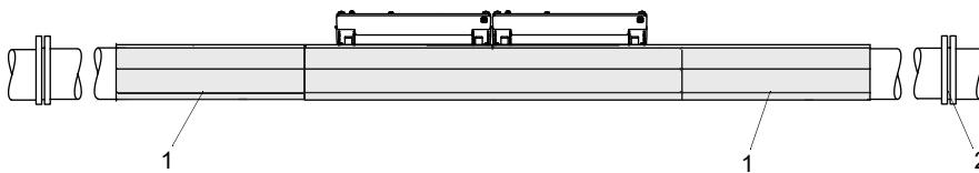
Fig. 6.9 : Atténuateurs acoustiques pour conduite et capteur en montage réflexion
