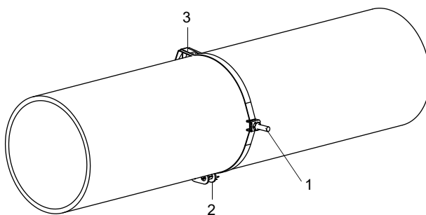
Fig. 6.50 : Bande de serrage avec pince et ressort métallique sur la conduite
