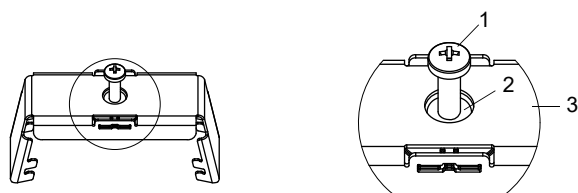
Fig. 6.64 : Étrier à ressort
