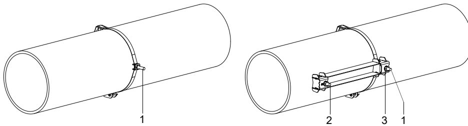
Fig. 6.32 : Rail fixé d'un côté à la conduite
