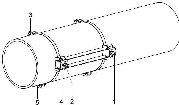
Fig. 6.33 : Rail sur la conduite
