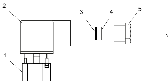
Fig. 7.27 : Montage du connecteur et du câble
