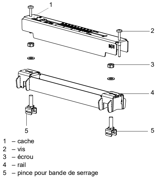
Fig. 6.21 : Démontage de la fixation Variofix L
