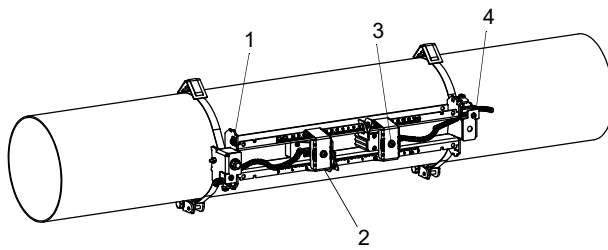
Fig. 6.65 : Capteurs dans le rail
