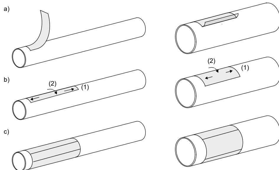
Fig. 6.11 : Fixation des atténuateurs acoustiques
