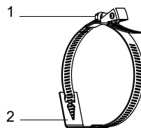
Fig. 6.52 : Bande de serrage avec fermoir rapide et ressort métallique
