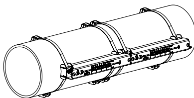
Fig. 6.20 : Fixation pour capteur Variofix L (montage réflexion)
