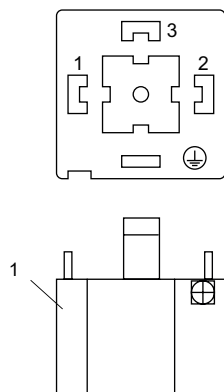
Fig. 7.26 : Brochage (connecteur)
