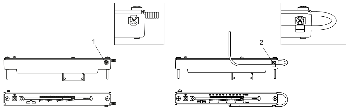
Fig. 6.41 : Fixation des câbles de capteurs
