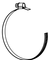
Fig. 6.47 : Fermoir de collier de serrage avec bande de serrage
