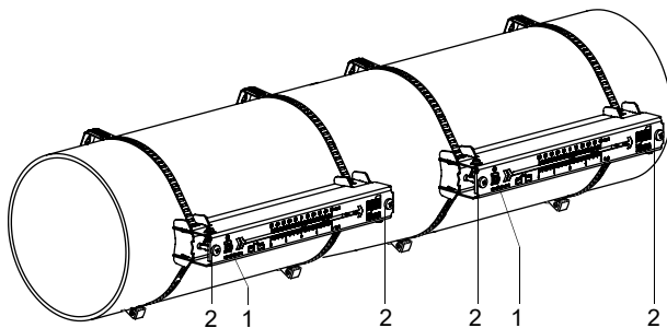
Fig. 6.42 : Variofix L avec capteurs sur la conduite
