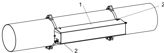
Fig. 6.66 : Variofix C avec capteurs sur la conduite
