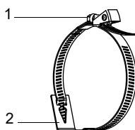
Fig. 6.35 : Bande de serrage avec fermeur rapide et ressort métallique
