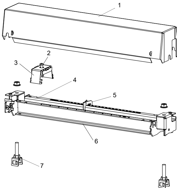
Fig. 6.46 : Démontage de la fixation Variofix C
