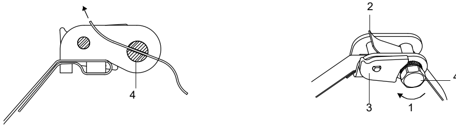
Fig. 6.37 : Fermeoir à cliquet avec bande de serrage
