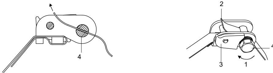
Fig. 6.62 : Fermeture à cliquet avec bande de serrage
