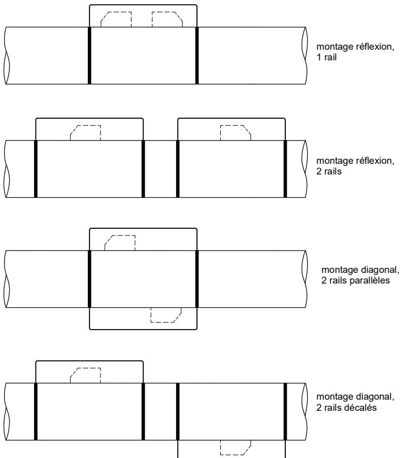
Fig. 6.15 : Disposition des capteurs dans les rails de montage
