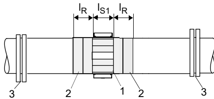
Fig. 6.13 : Diamètre extérieur de la conduite > 900 mm
