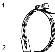
Fig. 6.60 : Bande de serrage avec fermoir rapide et ressort métallique
