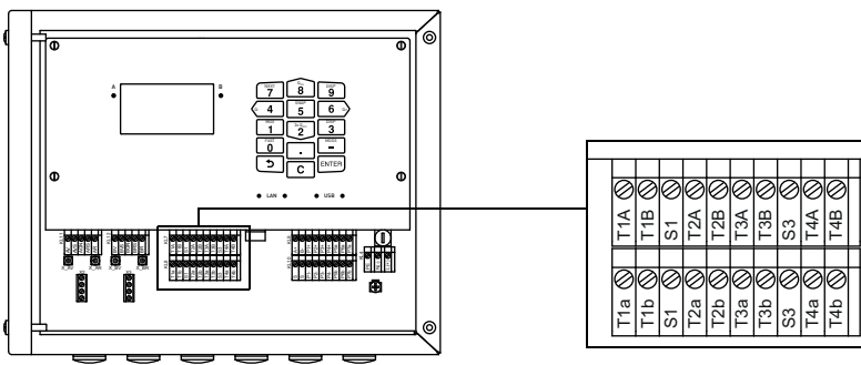
Fig. 7.30 : Raccordement des entrées au transmetteur
