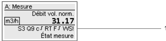
Fig. 9.5 : Affichage de la ligne d'état
