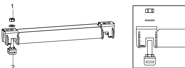
Fig. 6.31 : Rail avec pince pour bande de serrage
