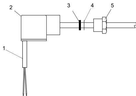
Fig. 7.24 : Montage du câble
