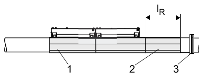
Fig. 6.12 : Diamètre extérieur de la conduite < 900 mm
