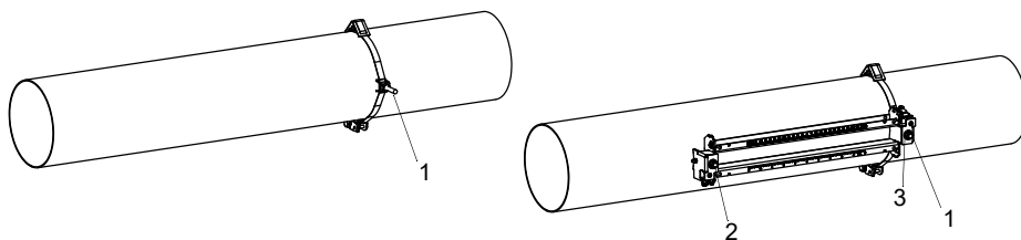
Fig. 6.57 : Rail fixé d'un côté à la conduite
