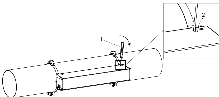
Fig. 6.67 : Retrait du cache
