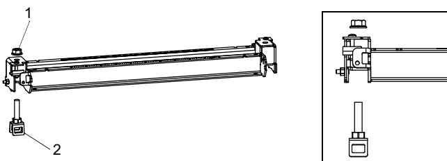
Fig. 6.56 : Rail avec pince pour bande de serrage
