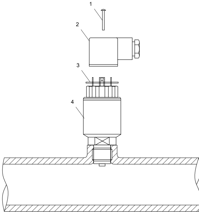
Fig. 7.28 : Fixation du connecteur
