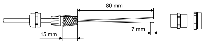
Fig. 7.32 : Câble préparé
