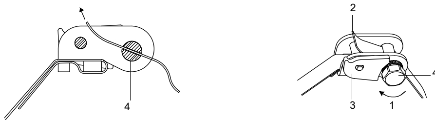
Fig. 6.55 : Fermeur à cliquet avec bande de serrage
