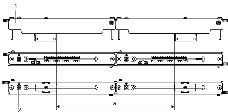
Fig. 6.40 : Réglage de l'écart entre les capteurs
