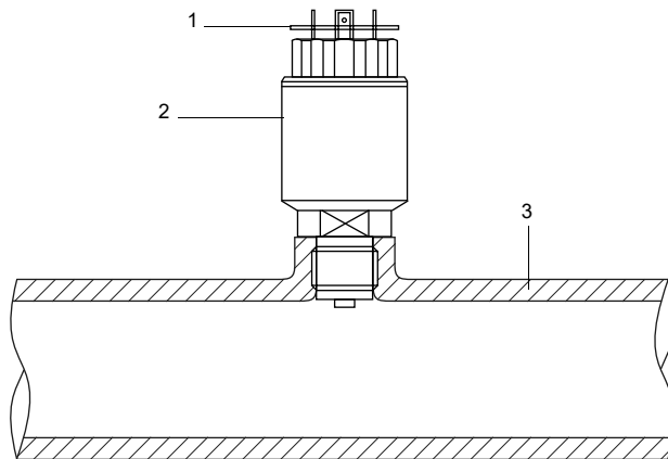
Fig. 6.76 : Transmetteur de pression monté
