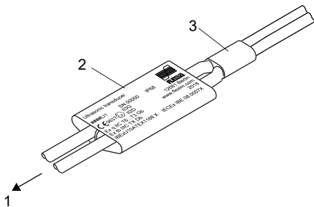
Fig. 6.18 : Plaquette signalétique au câble de capteurs
