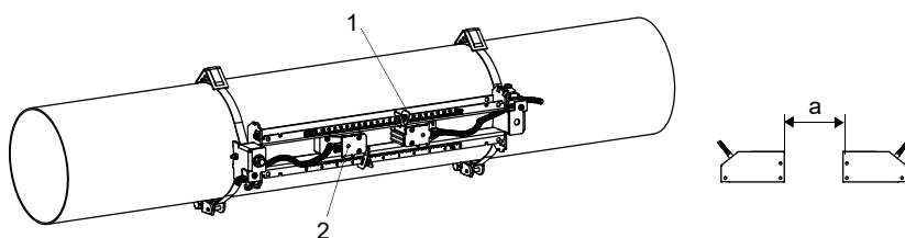
Fig. 6.63 : Capteurs dans le rail (étriers à ressort non représentés)
