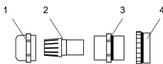
Fig. 7.31 : Presse-étoupe
