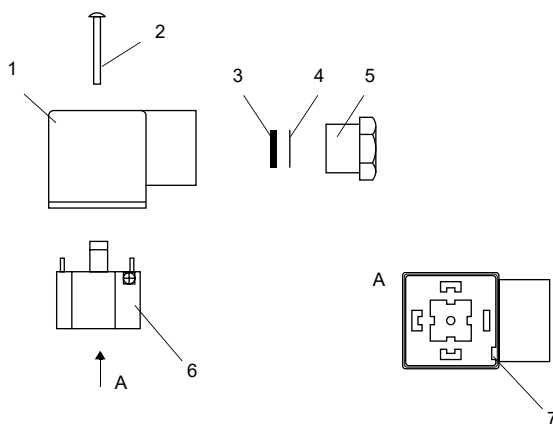
Fig. 7.23 : Connecteur démonté
