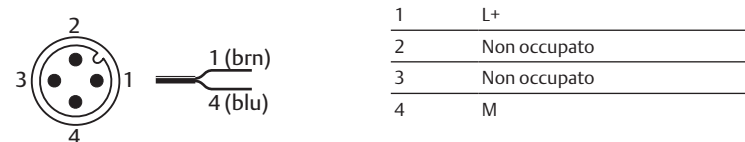
Fig. 1: Schema di collegamento sensore
