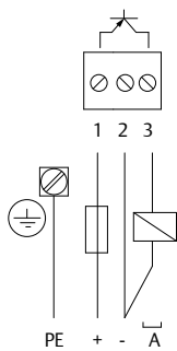
ábra 3-4: Tápellátás és jelkimenet (háromvezetékes PNP)
