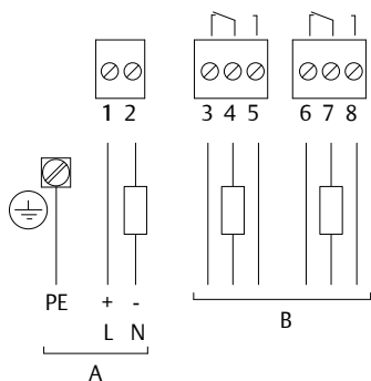
ábra 3-3: Tápellátás és jelkimenet (univerzális feszültségű verzió)
