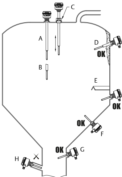
ábra 2-3: Helyes és helytelen szerelés
