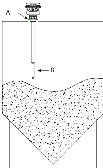
ábra 2-1: Mechanikai terhelés
