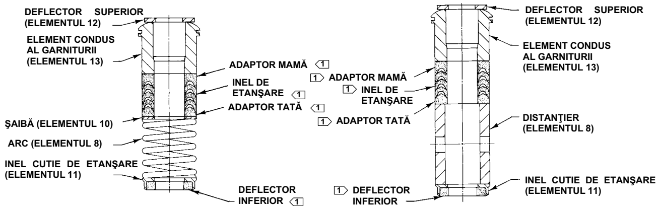
Figura 3. Configurații garnitură cu inel PTFE în V pentru capace plate și extensibile
