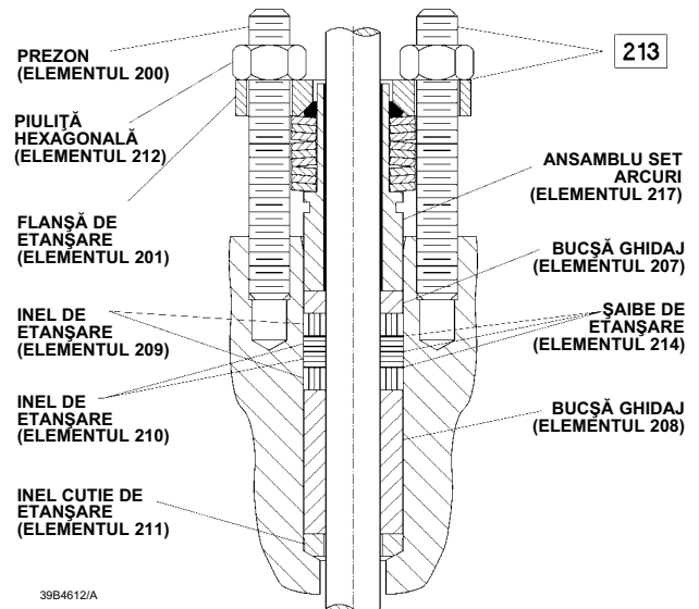
Figura 12. Sistem tipic ENVIRO-SEAL de etanșare cu garnitură ULF din grafit
