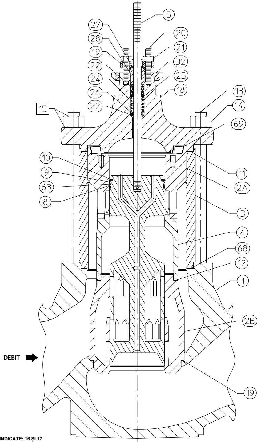
Figura 25. Ansamblu robinet NPS 8 cu DST în 3 trepte
