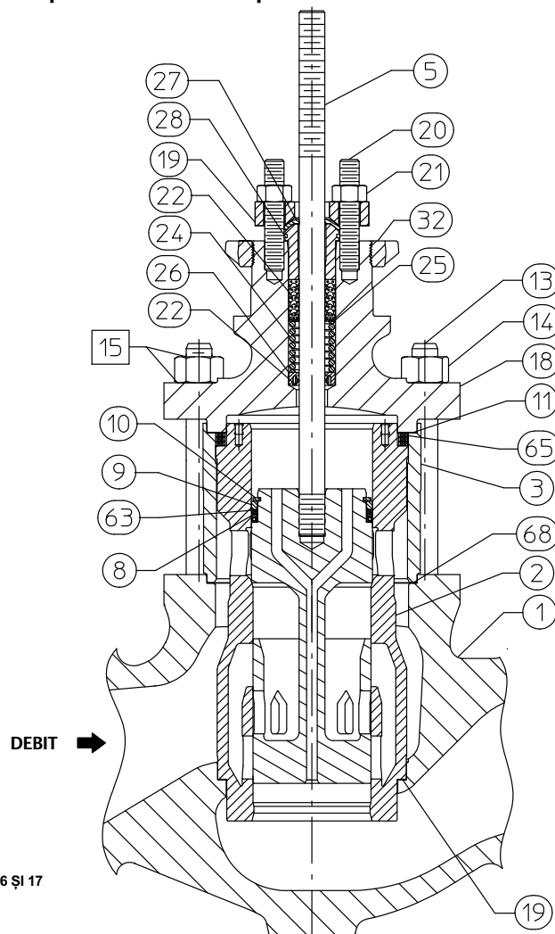
Figura 22. Ansamblu robinet tipic cu DST în 2 trepte
