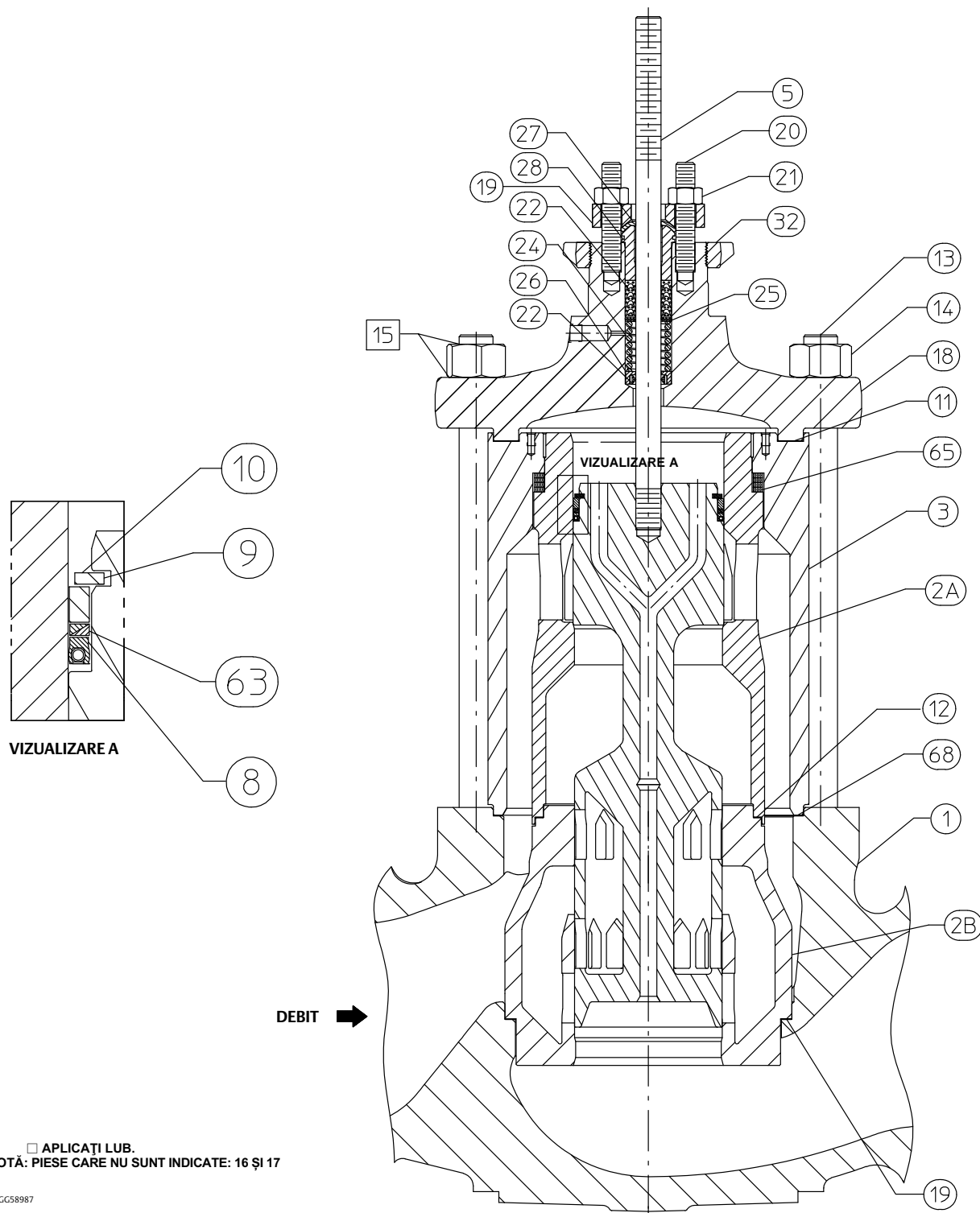
Figura 24. Ansamblu robinet NPS 6 cu DST în 3 trepte
