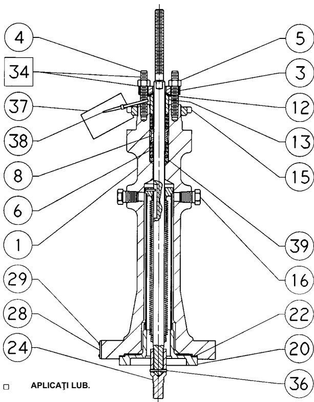
CAPAC DE ETANȘARE CU BURDUFURI ENVIRO-SEAL
