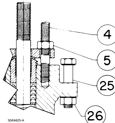
DETALIU PRINDERE DISPOZITIV DE ACȚIONARE CU BRIDE DE FIXARE DE 127 mm (5 IN.)
