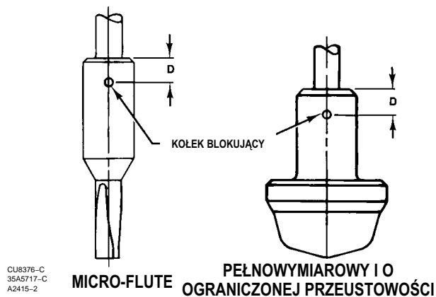
Ilustracja 10. Momenty sił dokręcających grzyb/trzpień lub grzyb/adapter i wymiana kołka blokującego
