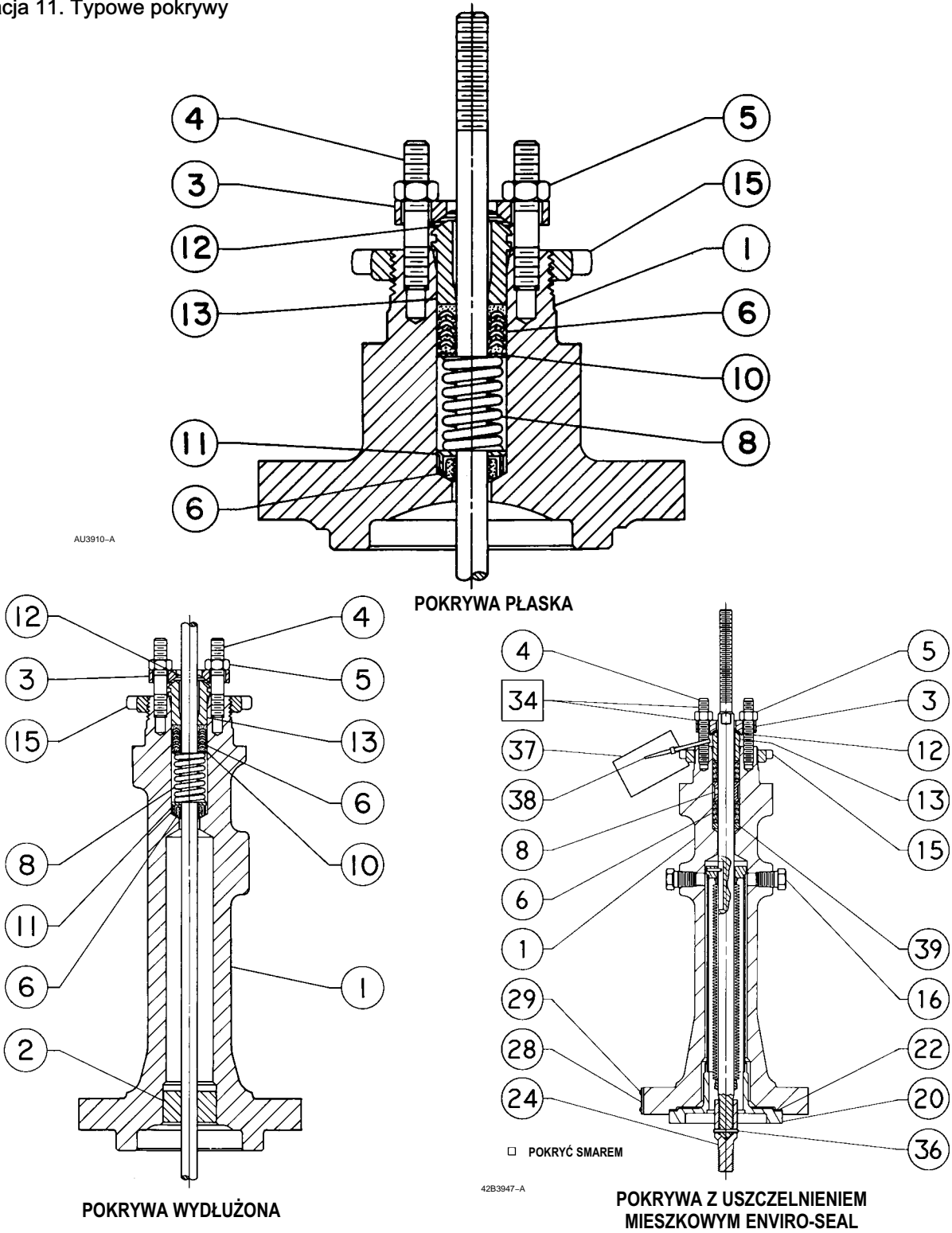
Ilustracja 11. Typowe pokrywy
