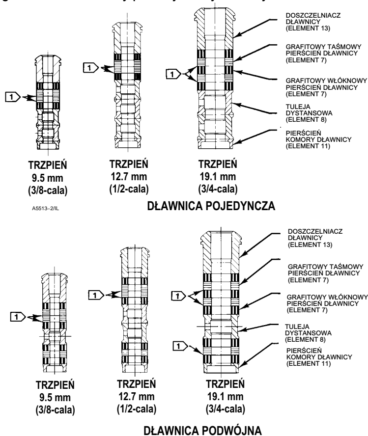
Ilustracja 5. Dławnice grafitowe do obudowy płaskiej lub wydłużonej
