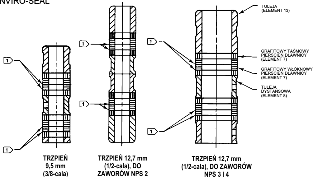
Ilustracja 15. Dławnice podwójne grafitowe taśmowo-włóknowe do pokryw z uszczelnieniem mieszkowym ENVIRO-SEAL
